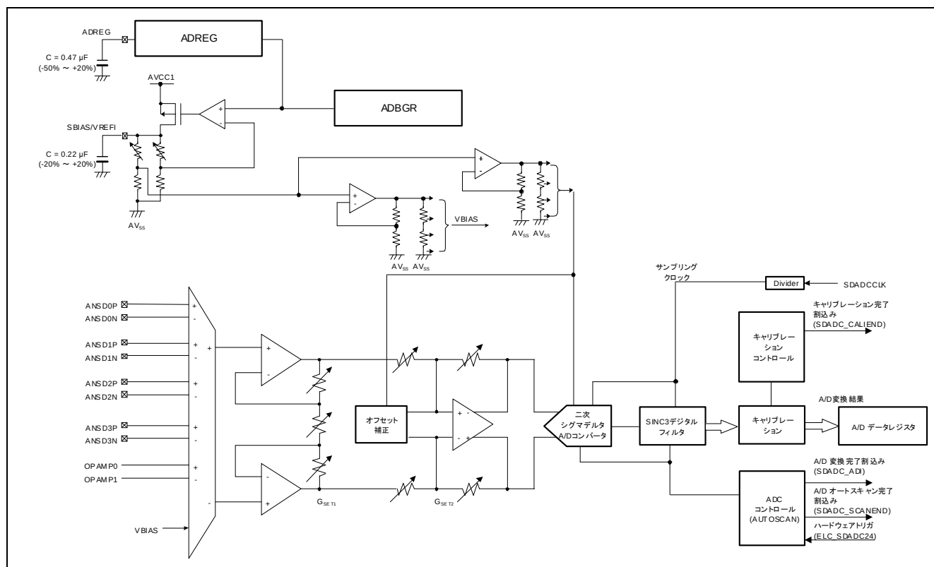
図 1 SDADC24 のブロック図
