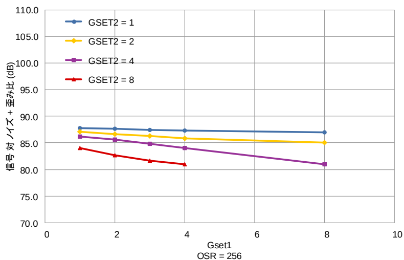
図 11 G_{SET1} に対する SINAD の依存性
