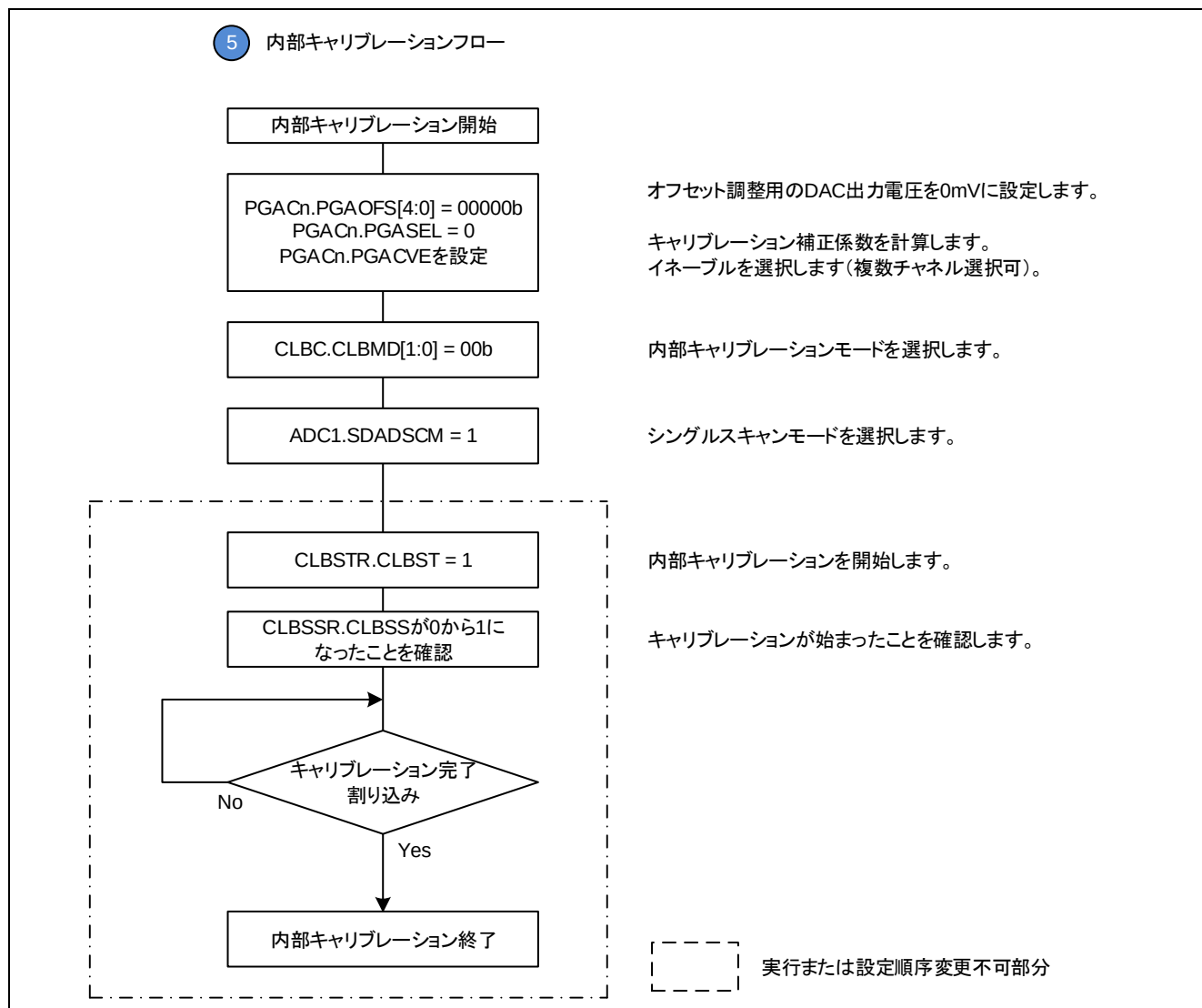
図 30 内部キャリブレーションフロー
