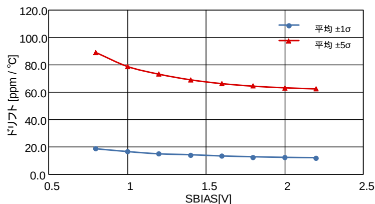
図 21 ドリフトと SBIAS の対比
