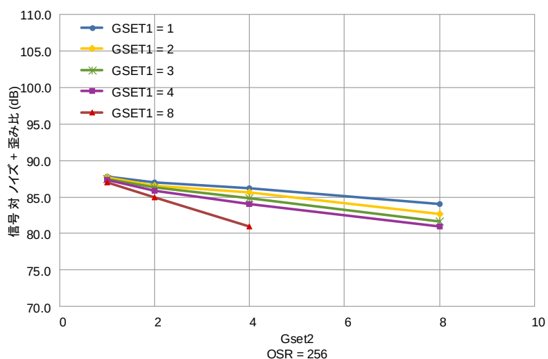
図 12 G_{SET2} に対する SINAD の依存性
