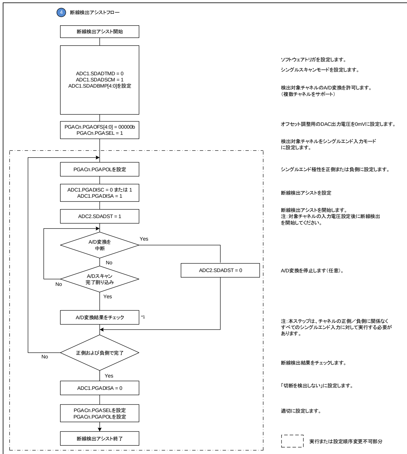
図 29 断線検出アシストフロー
