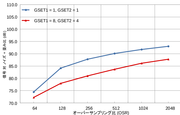
図 8 SINAD と OSR の対比
