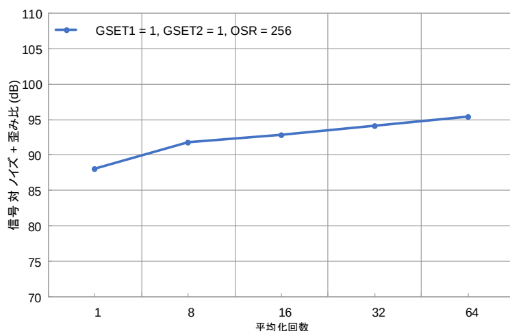
図 20 SINAD と平均化回数の対比
