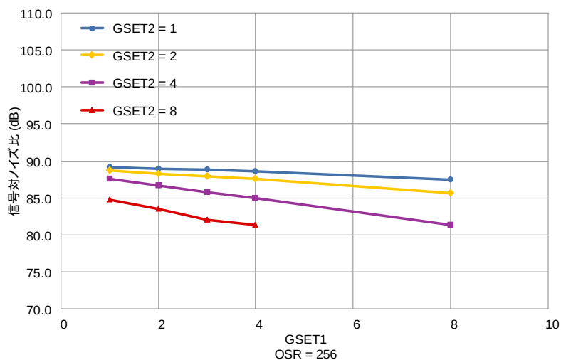
図 9 G_{SET1} に対する SNR の依存性
