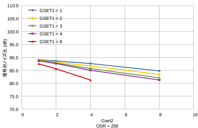
図 10 G_{SET2} に対する SNR の依存性
