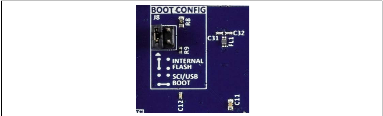
図 2 ボード起動時に動作モードを設定するジャンパー J8 の配置場所
