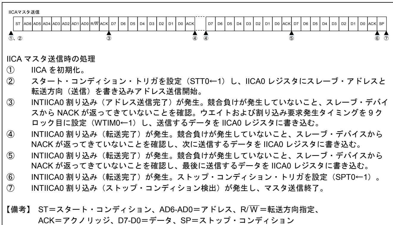
図 2.2 IICA マスタ送信の処理 (タイミング図)
