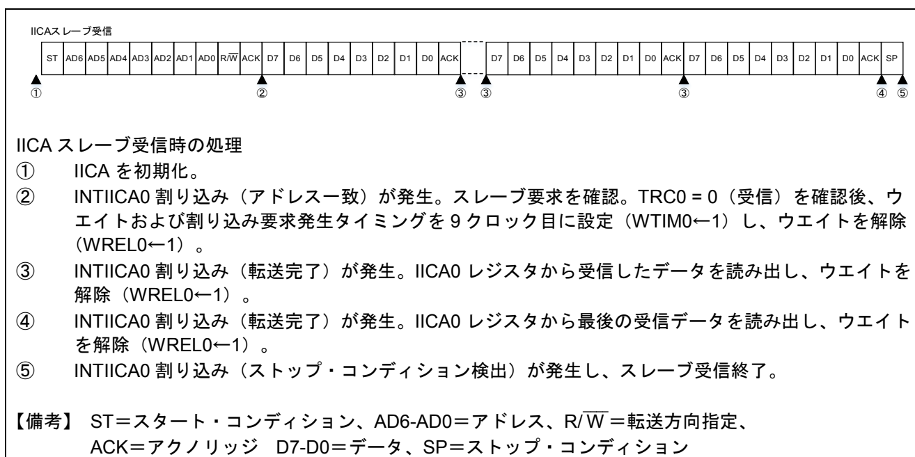
図 2.5 IICA スレーブ受信の処理（タイミング図）
