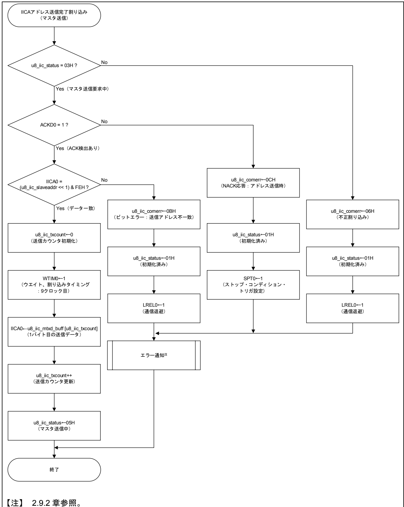
図 2.14 IICA アドレス送信完了割り込み処理（マスタ送信）
