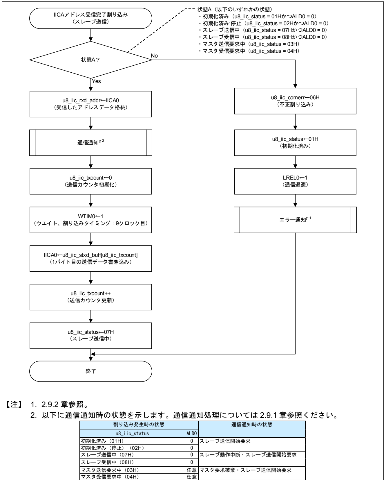
図 2.16 IICA アドレス受信完了割り込み処理（スレーブ送信）
