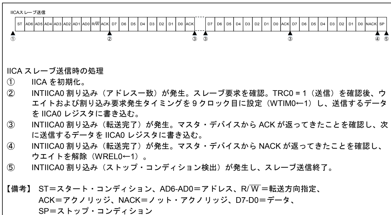
図 2.4 IICA スレーブ送信の処理（タイミング図）
