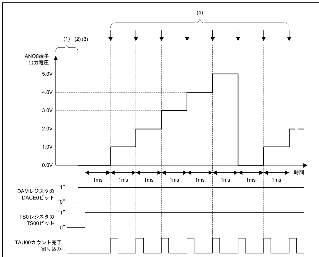
図4.1 タイミング図
