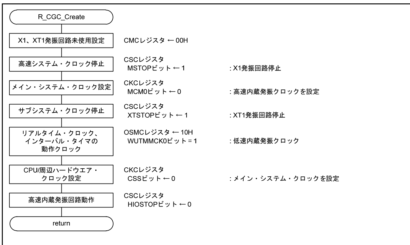
図4.5 CPU クロック初期設定
