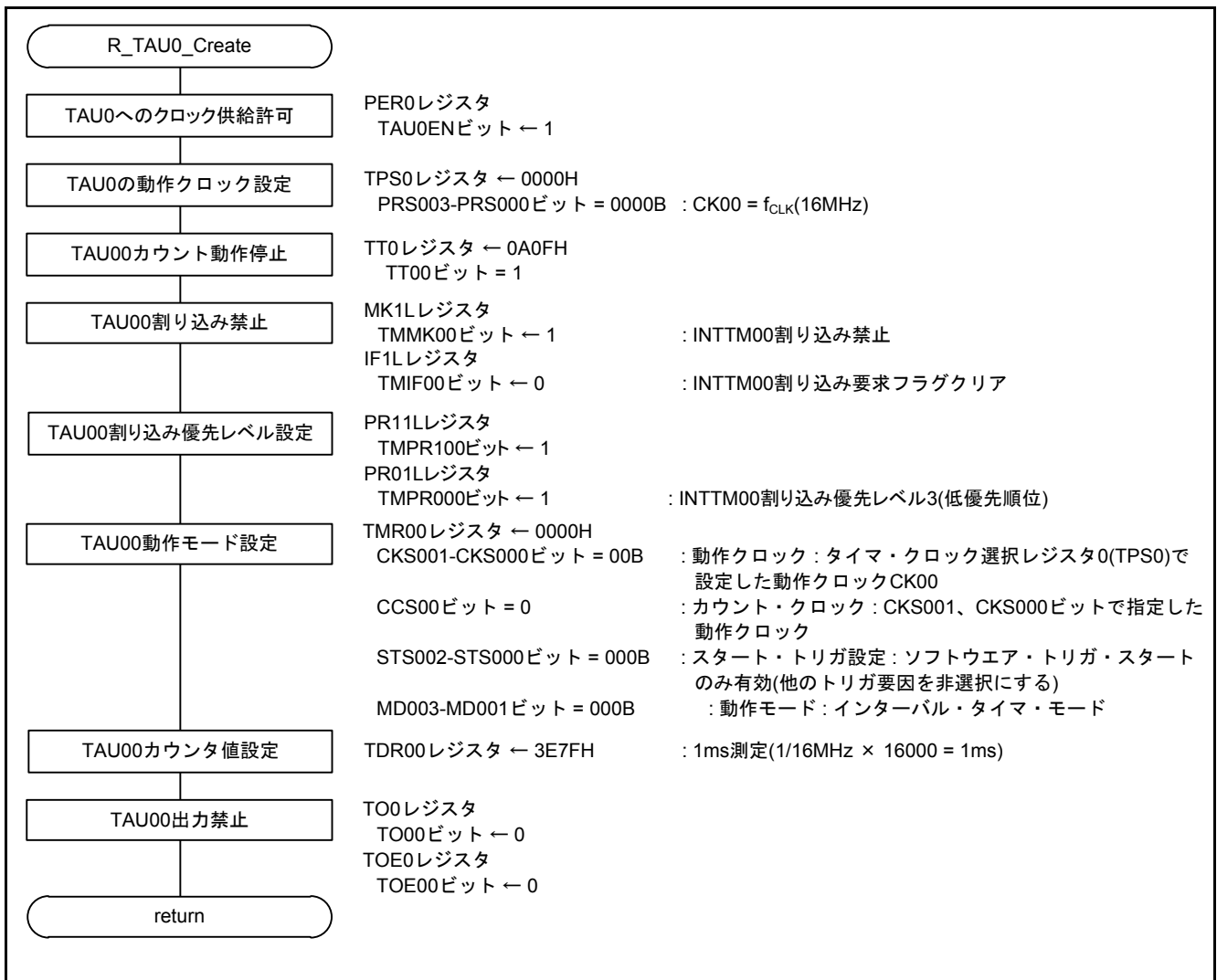
図4.6 TAU0 初期設定
