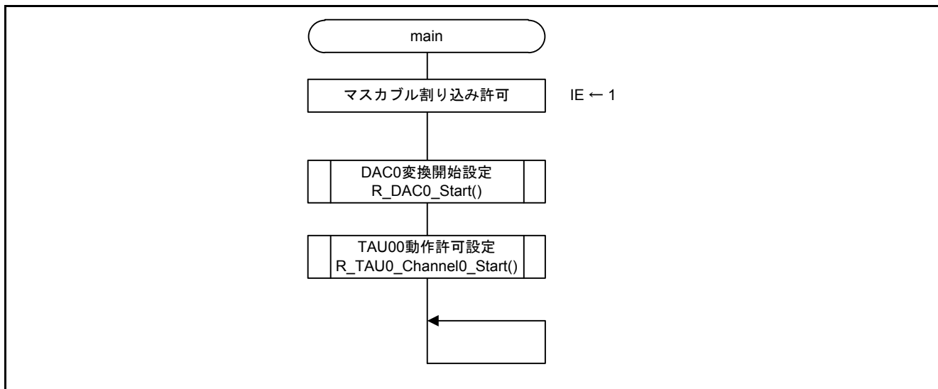
図4.8 メイン処理
