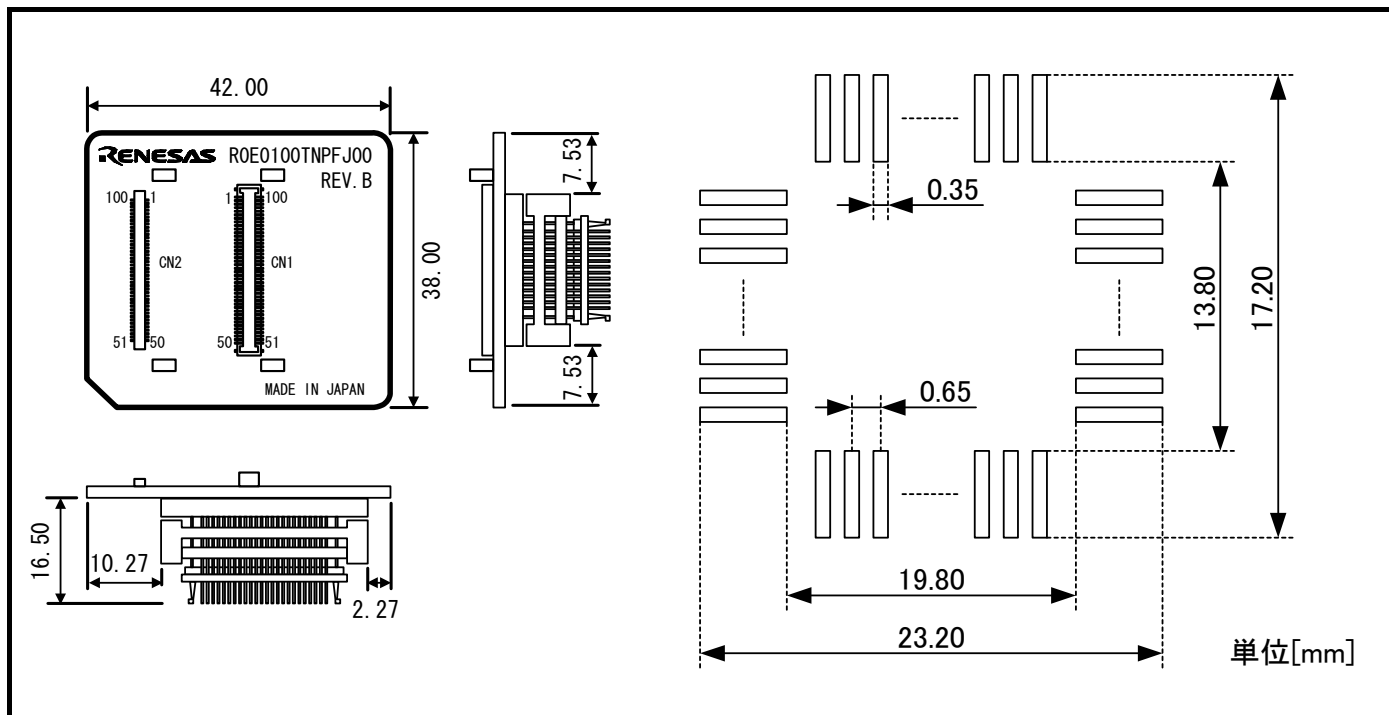
図7.3 R0E0100TNPfJ00ユーザーシステム接続部の寸法図および参考フットパターン
