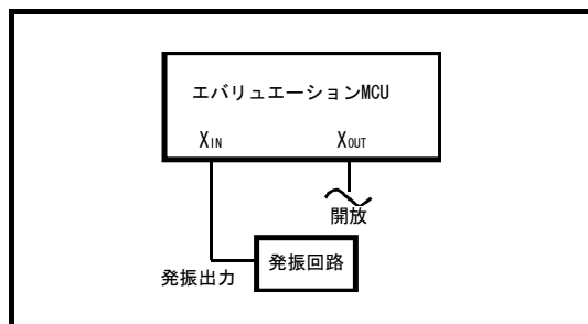
図2.8 ユーザシステム上発振回路の使用
