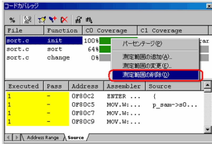
図5.90 [コードカバレッジ] ウィンドウ
