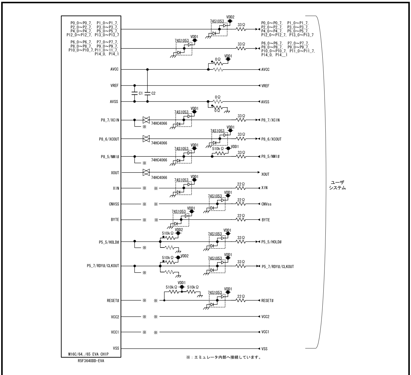
図7.1 R0E530640MCU00の接続図(一部)
