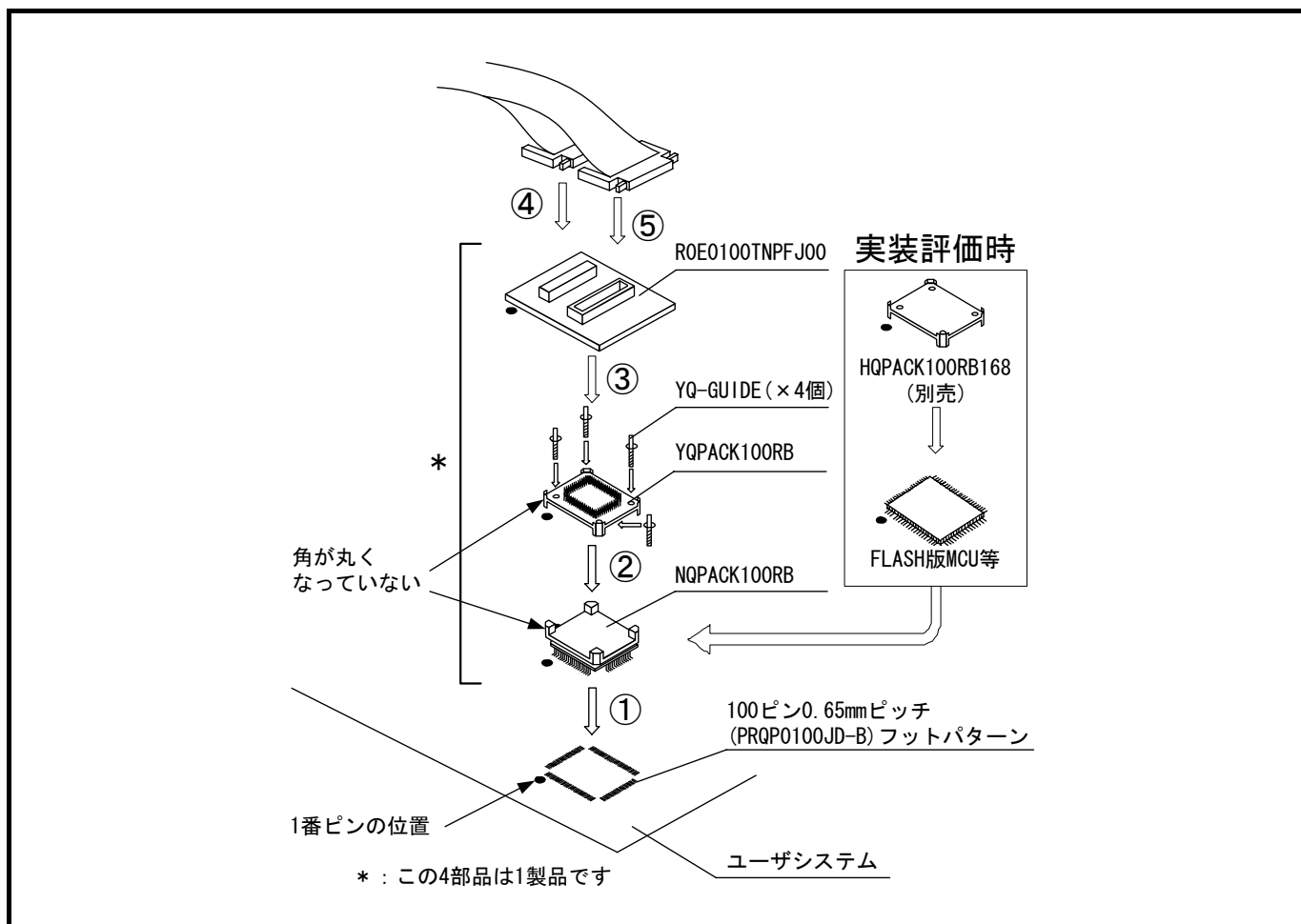
図2.11 100ピン0.65mmピッチフットパターンへの接続
