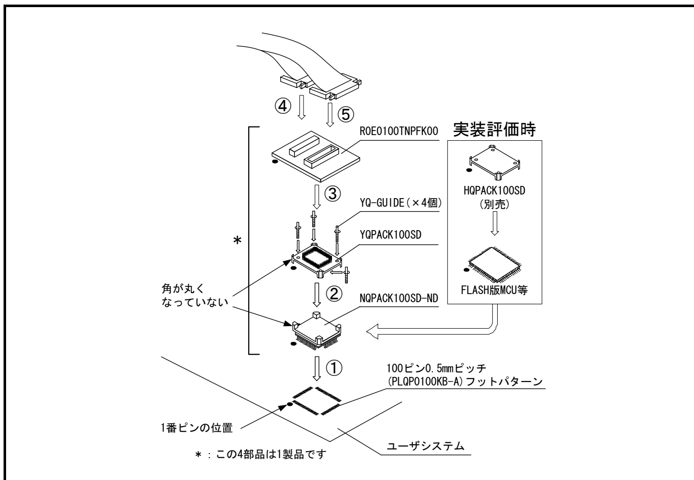
図2.12 100ピン0.5mmピッチフットパターンへの接続
