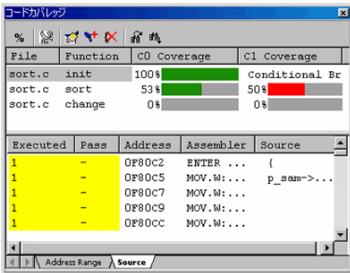
図5.86 [コードカバレッジ] ウィンドウ
