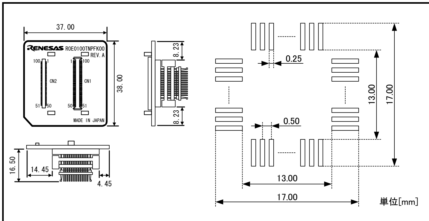
図7.4 R0E0100TNPFK00ユーザーシステム接続部の寸法図および参考フットパターン
