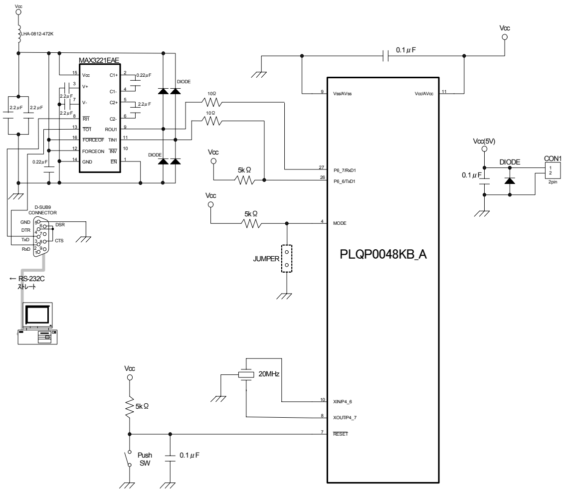
図 2 RS-232C ケーブルを使用した回路例
