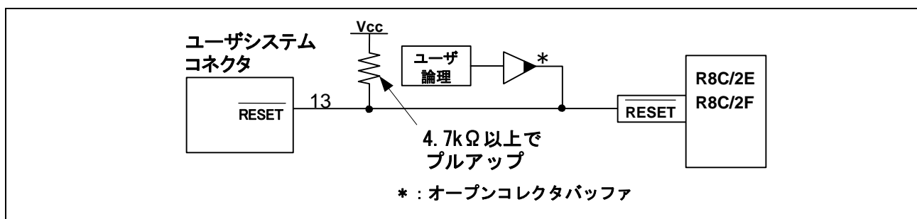
図 5.3 リセット回路例
