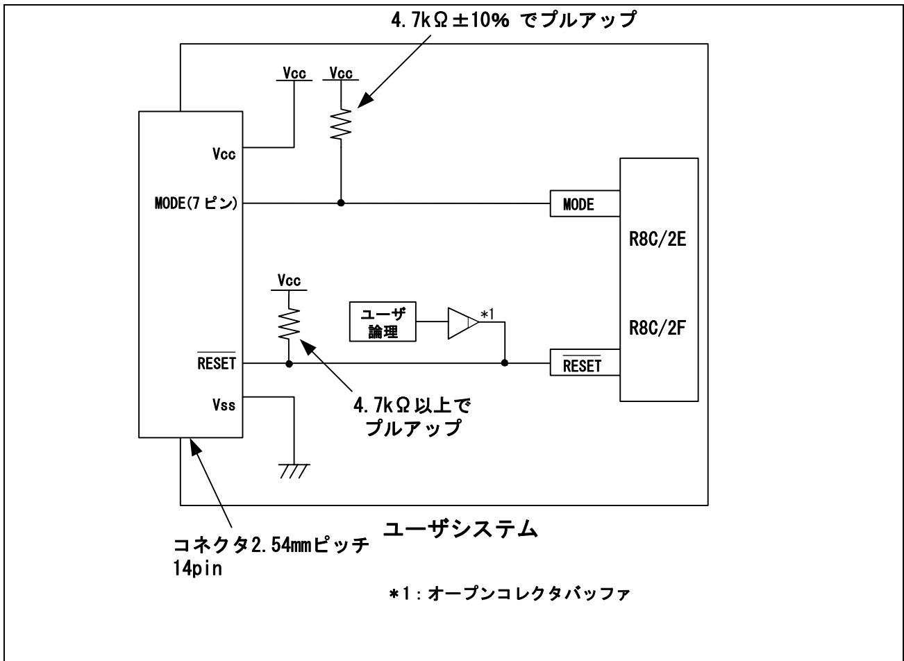
図 5.1 E8 の接続例
