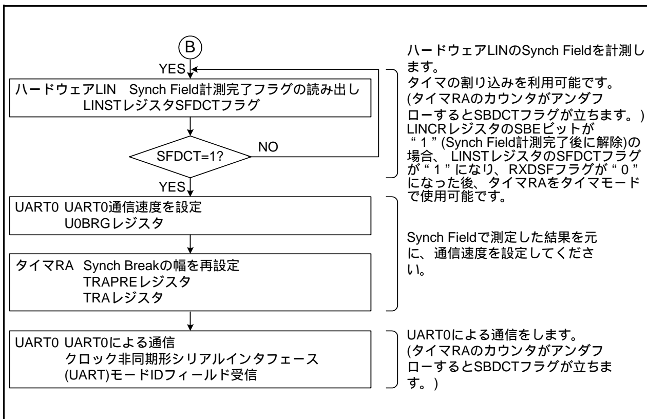
図26.8 ヘッドフィールド受信フローチャート例(3)
