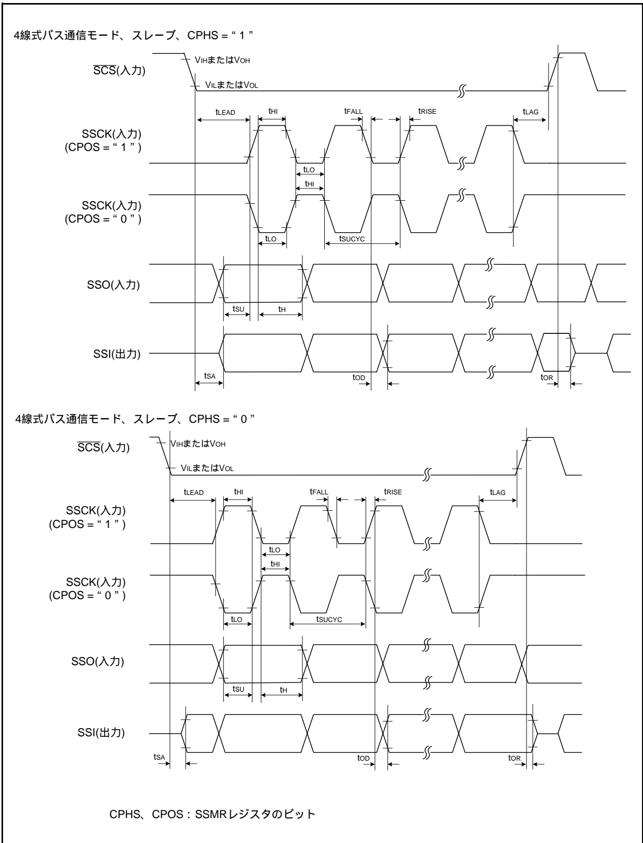
図33.5 チップセレクト付クロック同期形シリアルI/Oの入出力タイミング(スレーブ)
