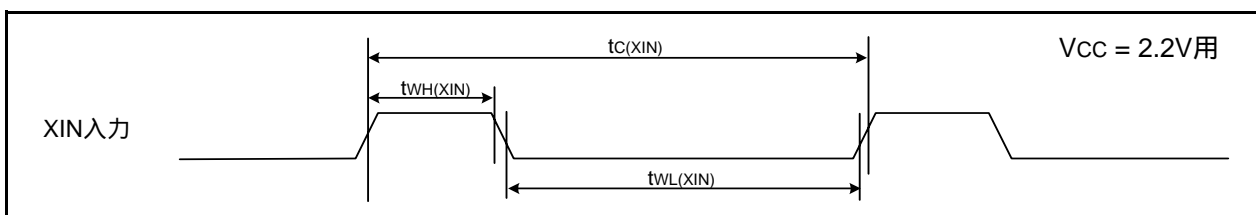
図33.16 V_{CC} = 2.2V 時のXIN入力、XCIN入力タイミング
