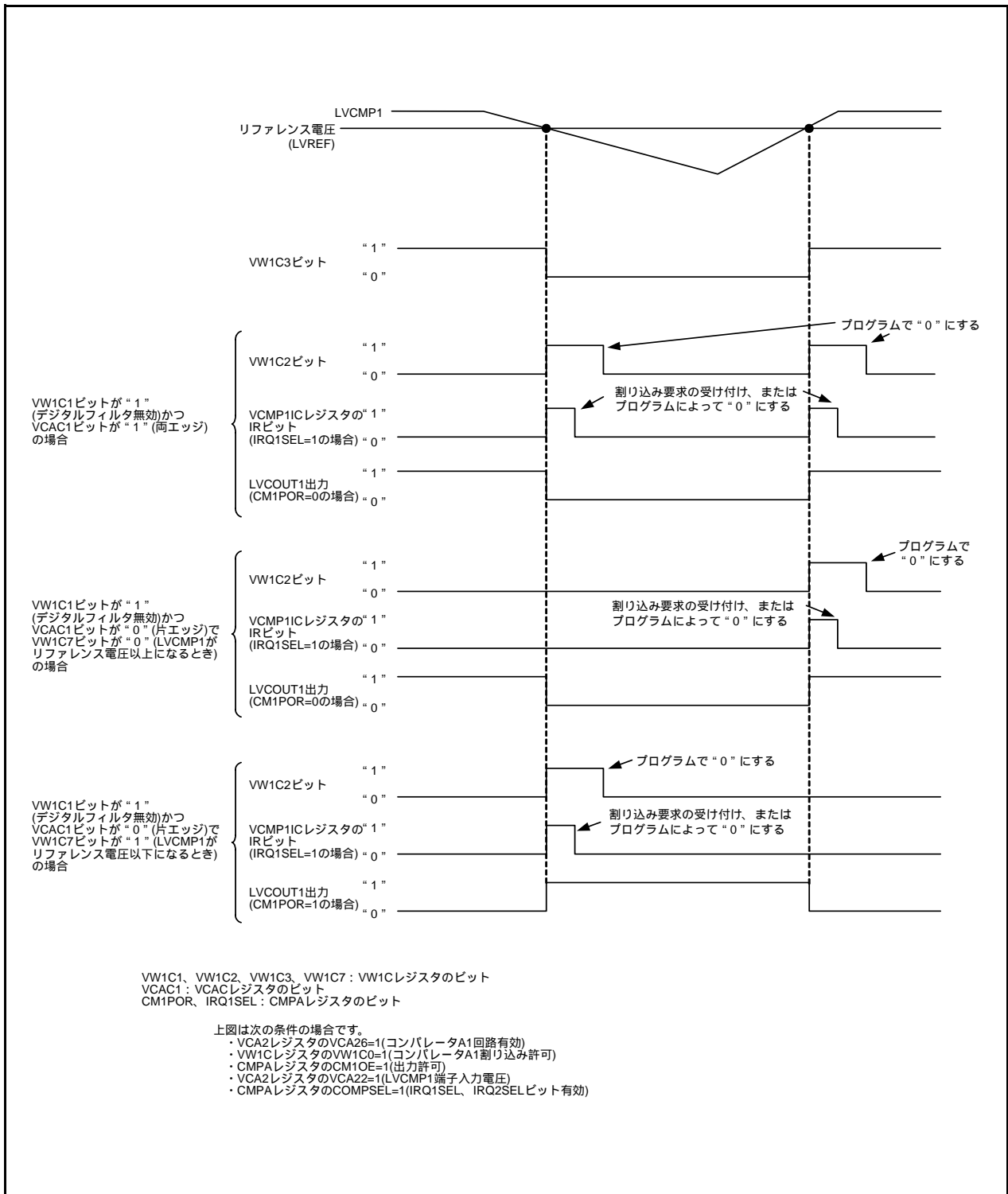
図 29.3 コンパレータA1動作例(デジタルフィルタ無効の場合)
