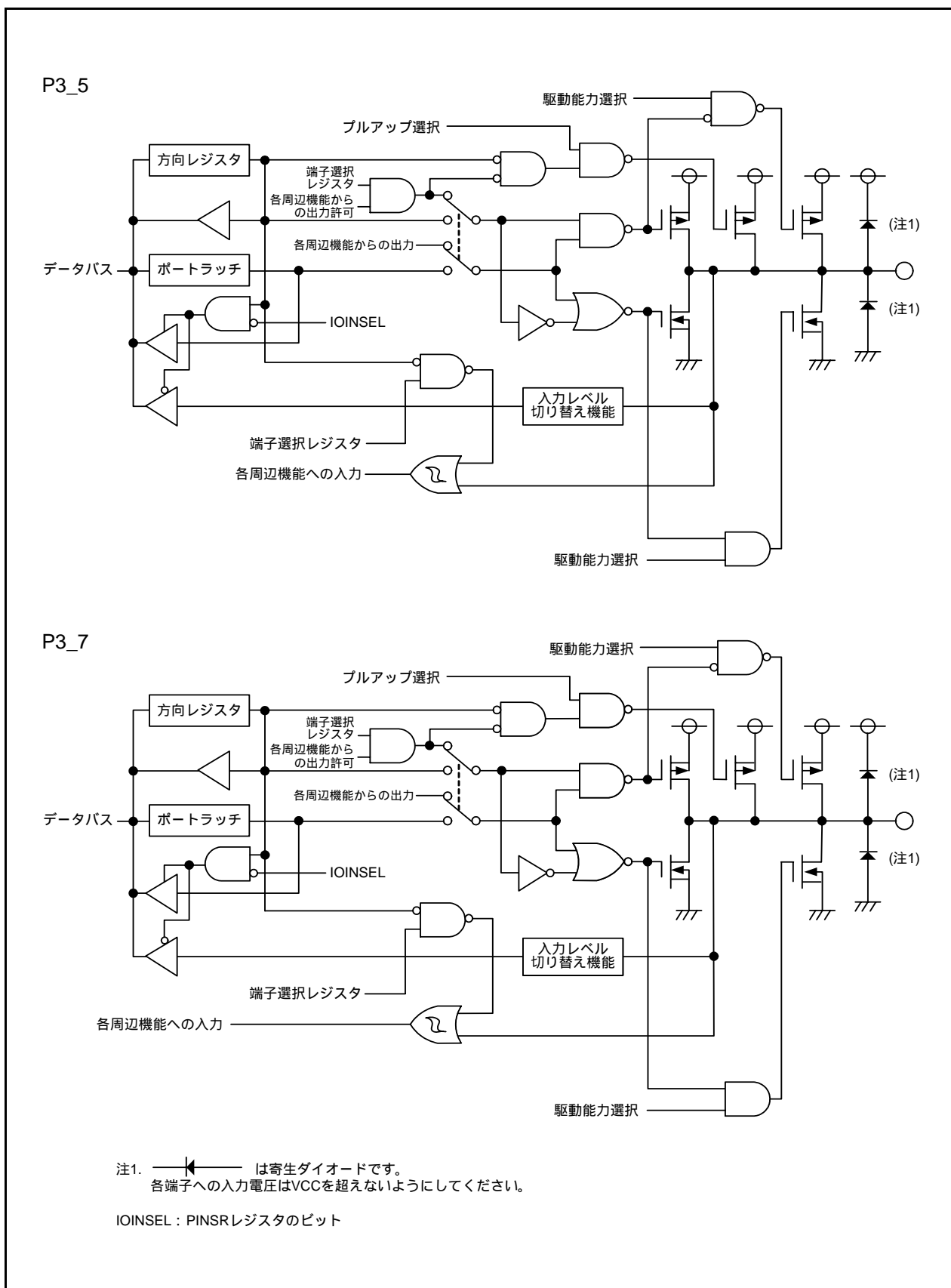
図7.6 I/Oポートの構成(7)
