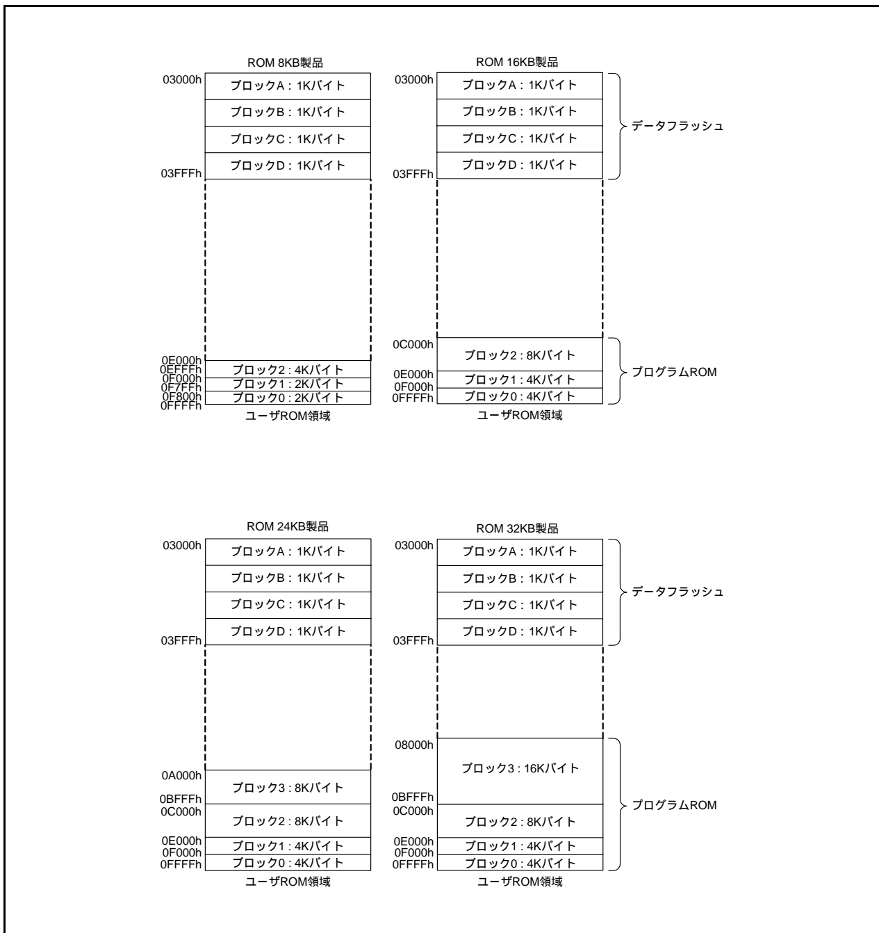
図 31.1 R8C/3GAグループのフラッシュメモリのブロック図
