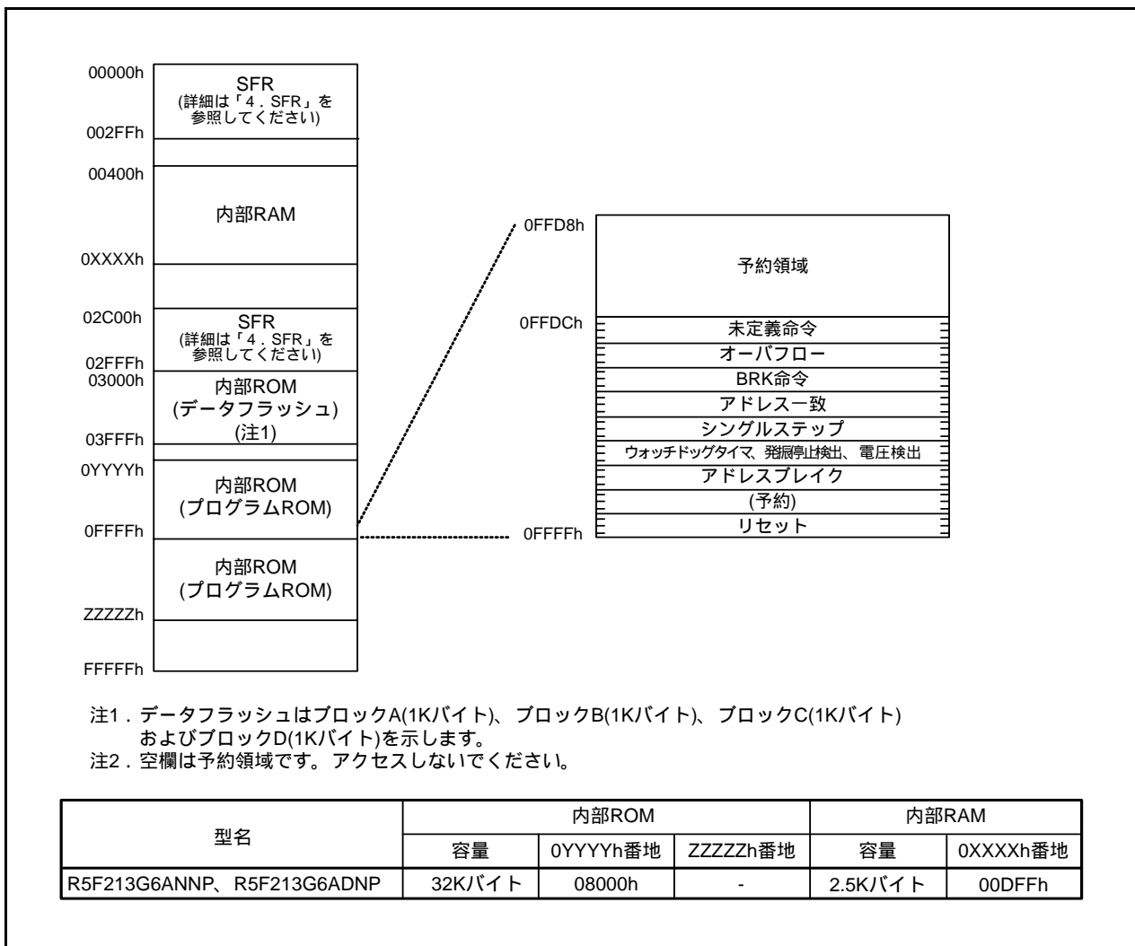
図3.1 R8C/3GAグループのメモリ配置図
