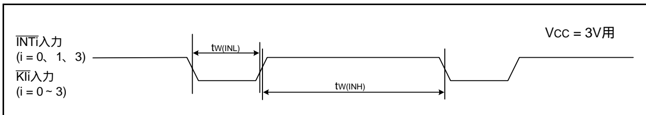
図33.15 Vcc = 3V時の外部割り込み \overline{INTi} およびキー入力割り込み \overline{Kli} 入力タイミング
