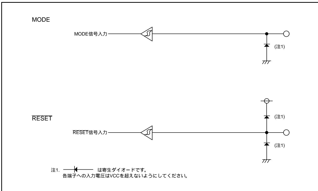
図7.9 端子の構成
