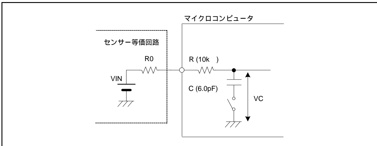
図27.10 アナログ入力端子と外部センサーの等価回路例
