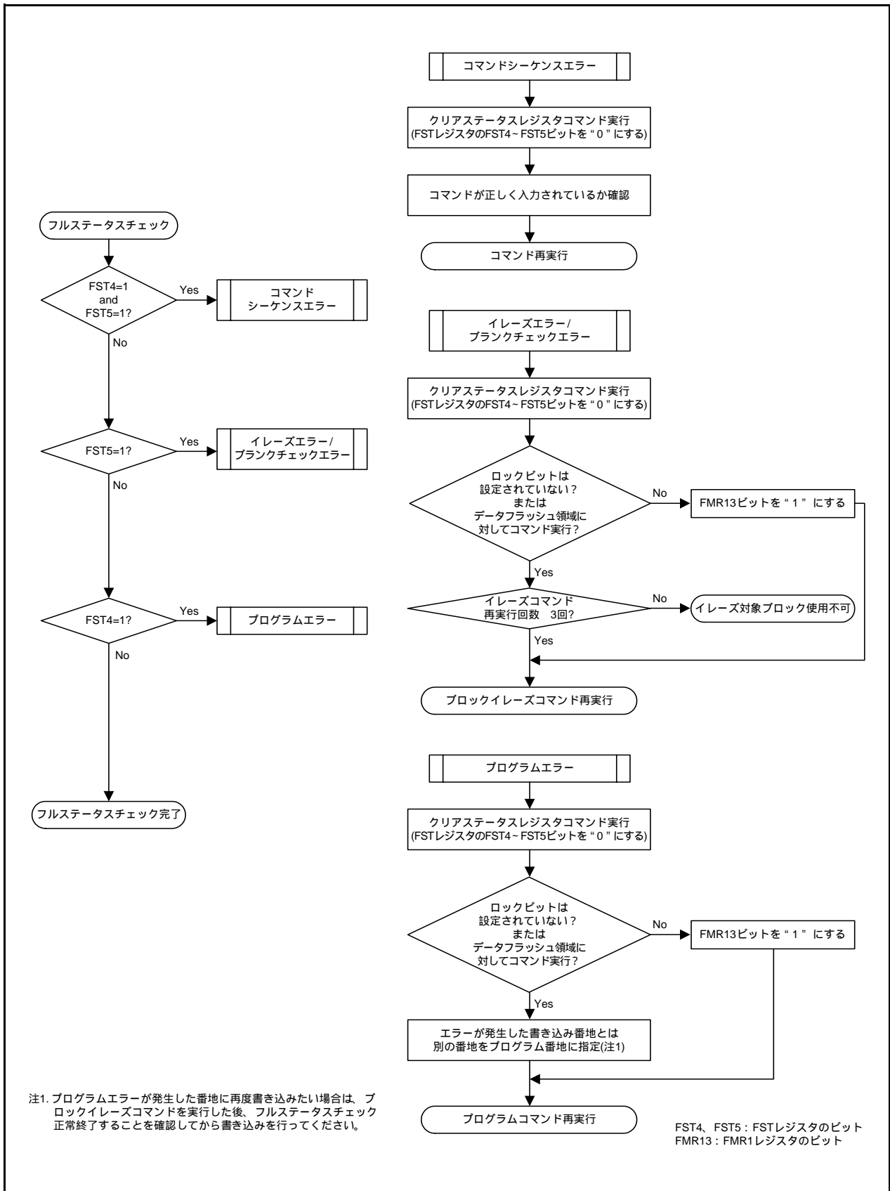
図 31.15 フルステータスチェックフローチャート、各エラー発生時の対処方法
