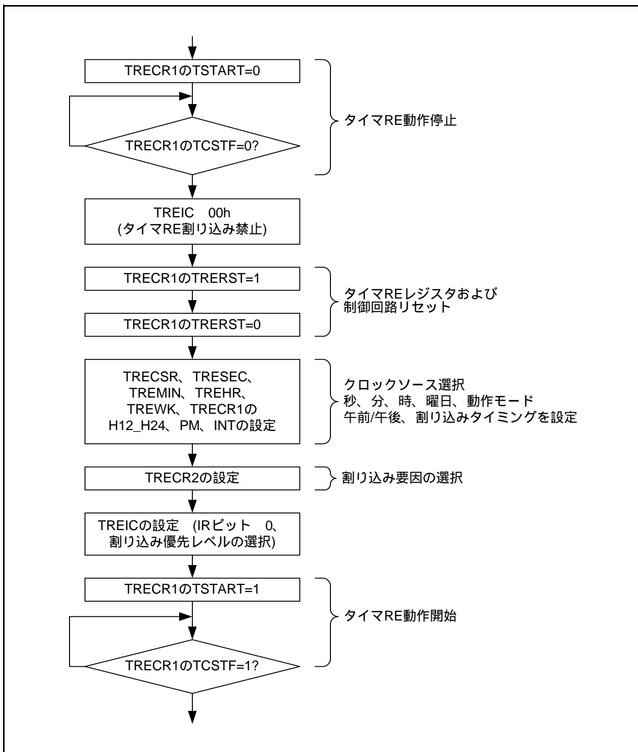
図 34.2 リアルタイムクロックモード時の設定例
