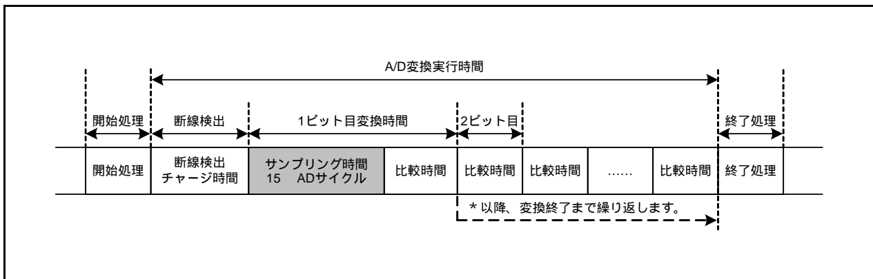
図 27.2 A/D変換タイミング図
