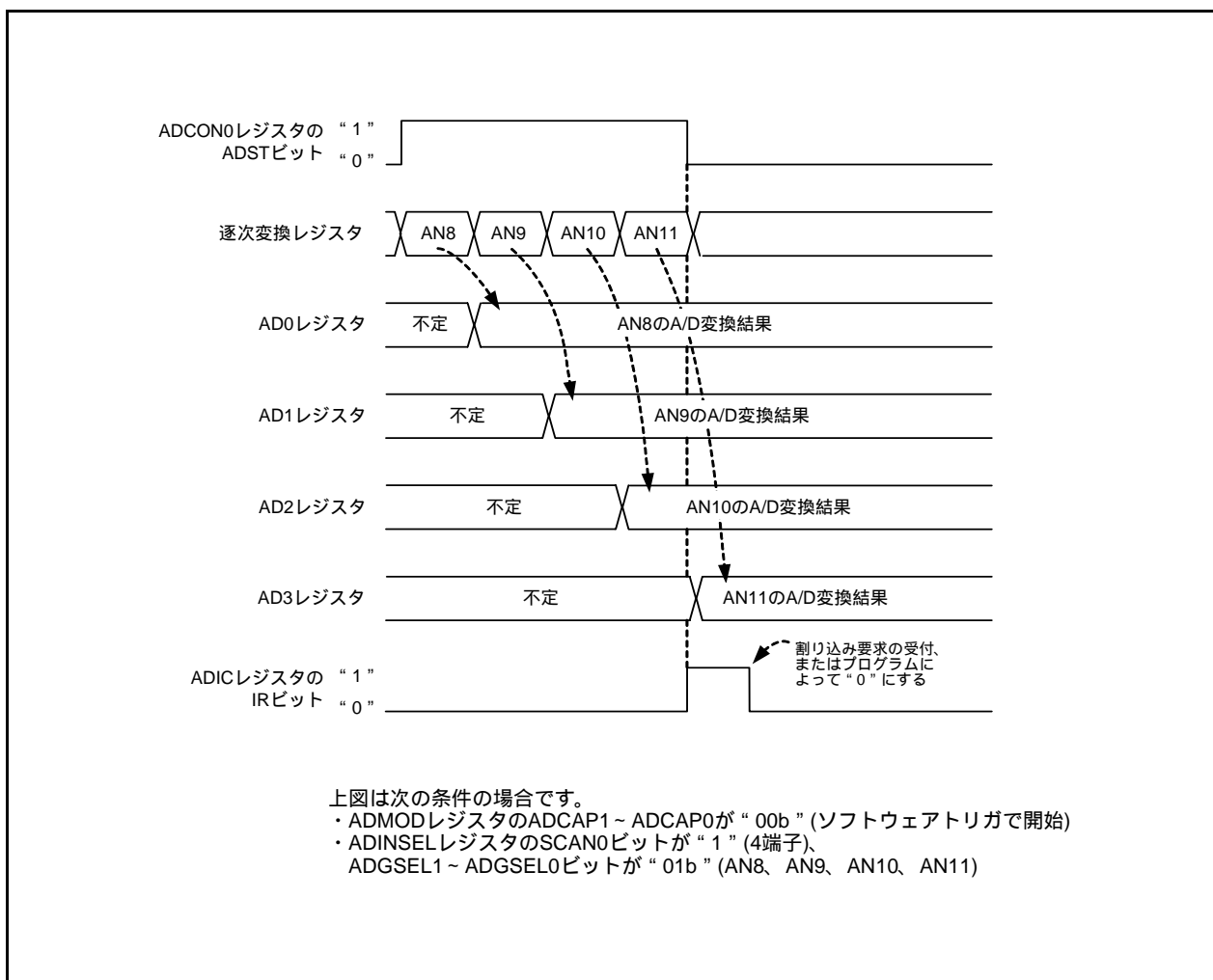
図 27.8 単掃引モード時の動作例
