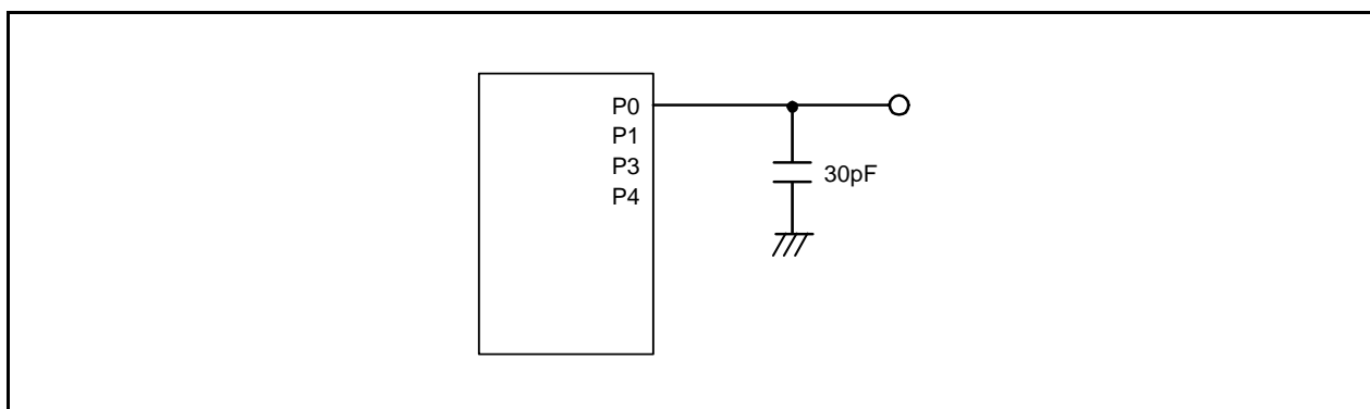
図33.1 ポートP0、P1、P3、P4のタイミング測定回路
