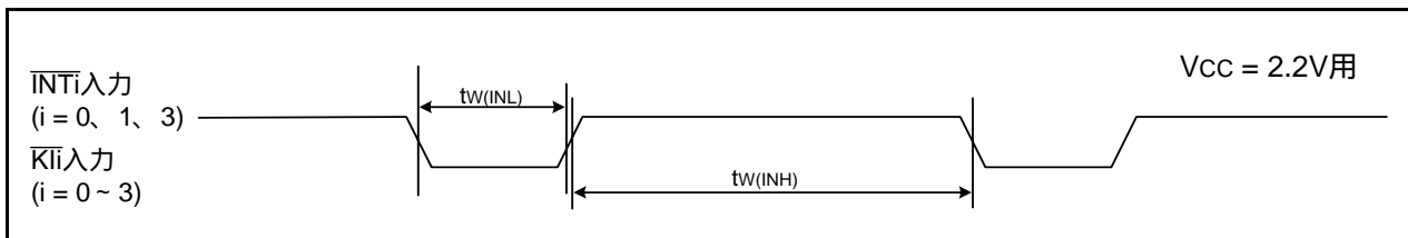
図33.19 Vcc = 2.2V時の外部割り込みINTiおよびキー入力割り込みKli入力タイミング
