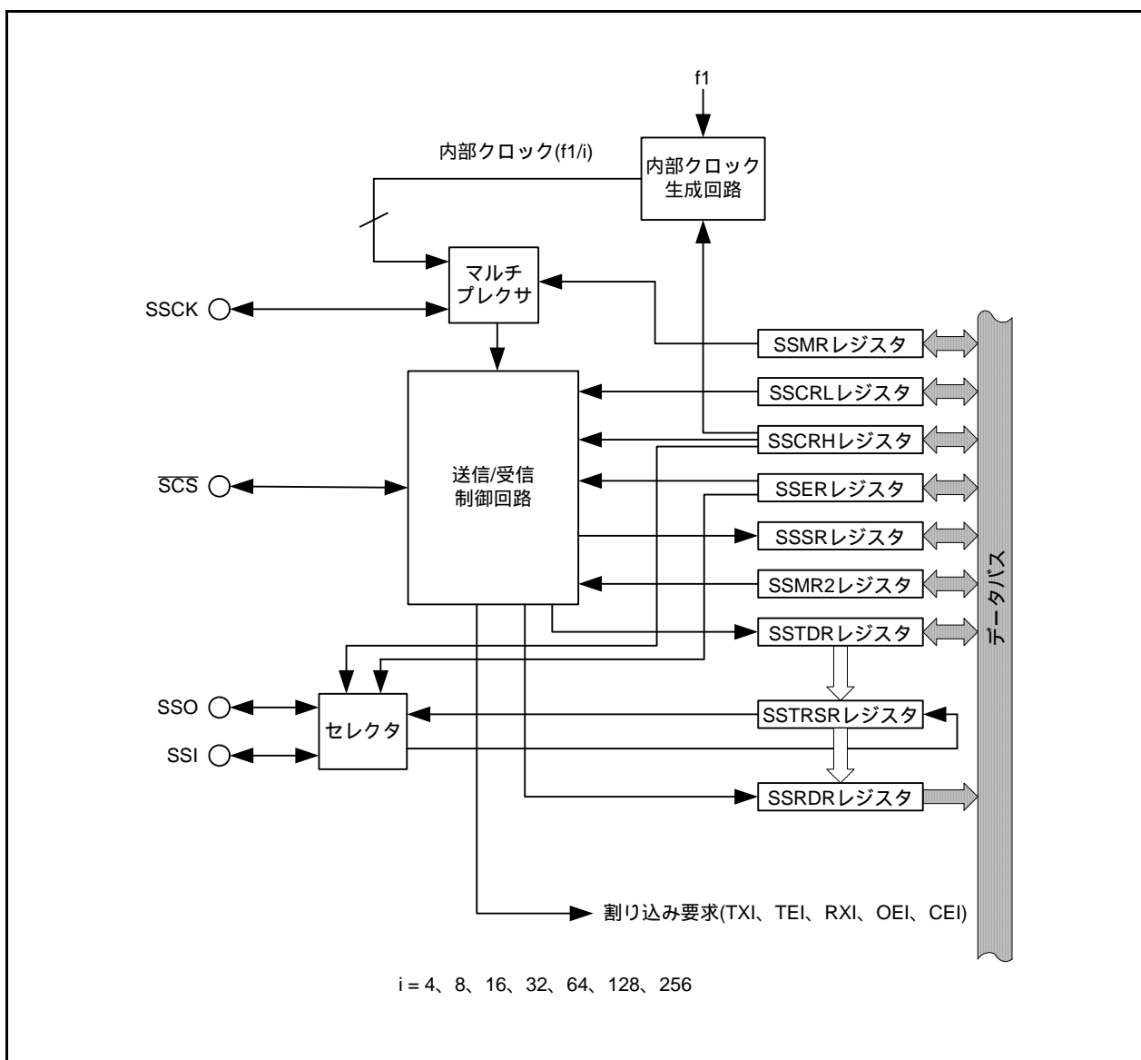
図 24.1 シンクロナスシリアルコミュニケーションユニットブロック図
