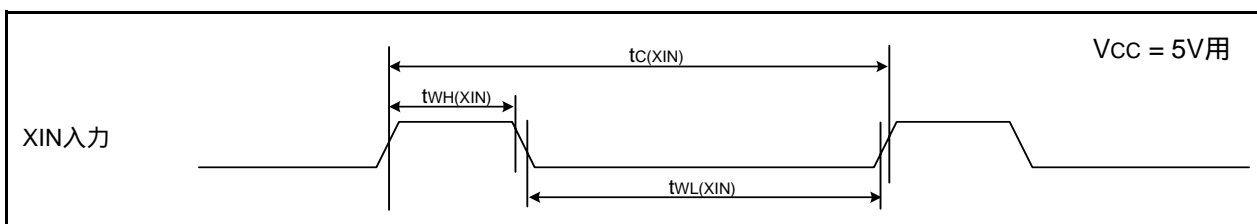
図33.8 V_{CC} = 5V 時のXIN入力、XCIN入力タイミング
