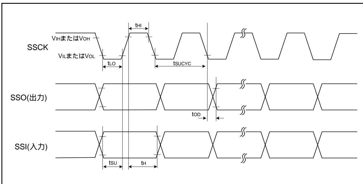
図33.6 チップセレクト付クロック同期形シリアルI/Oの入出力タイミング(クロック同期式通信モード)
