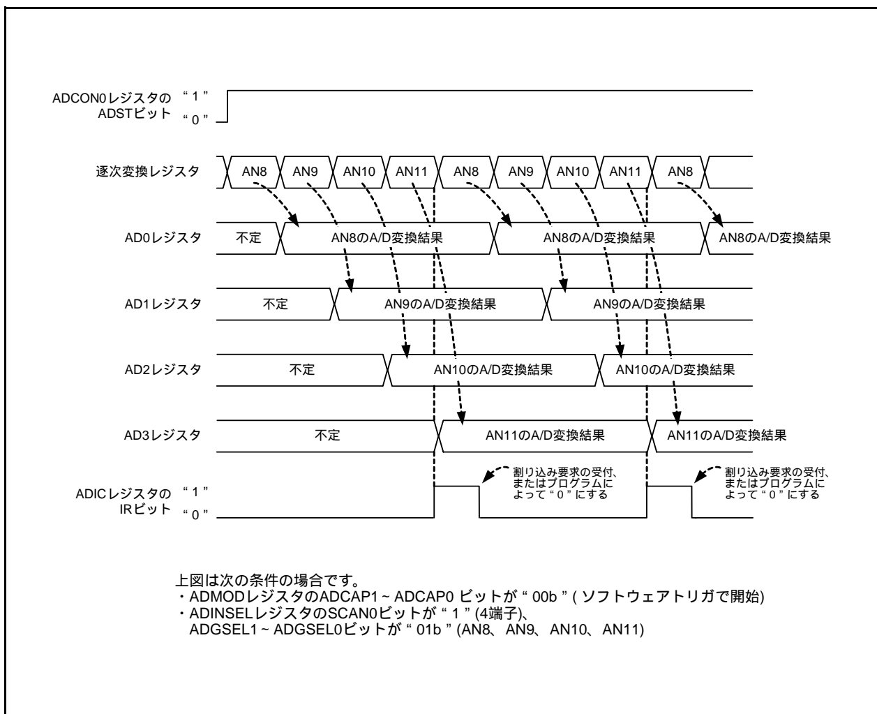
図 27.9 繰り返し掃引モード時の動作例
