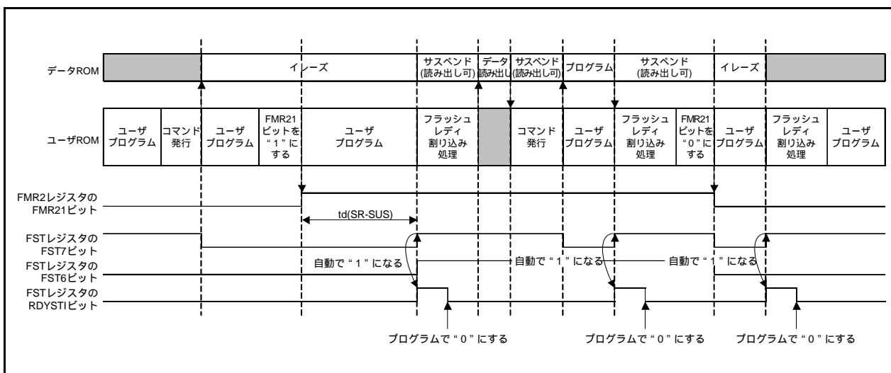
図 31.2 サスペンド動作に関するタイミング
