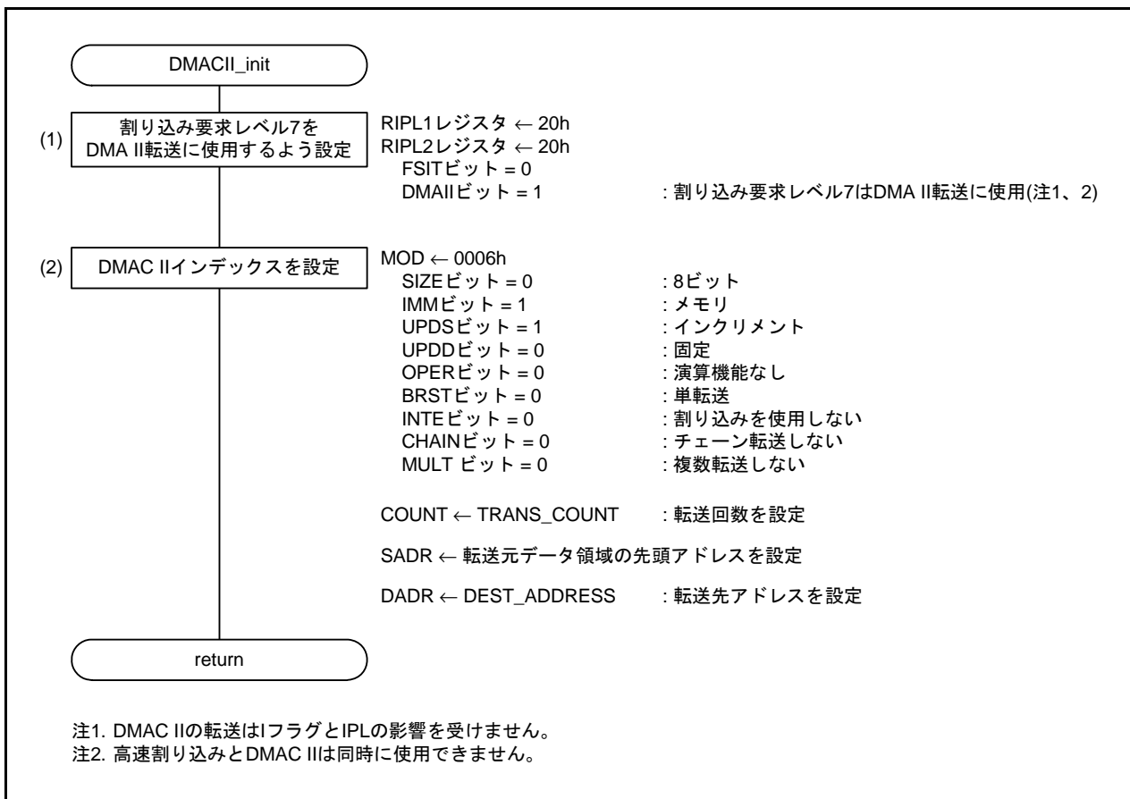
図 5.6 DMAC II初期設定
