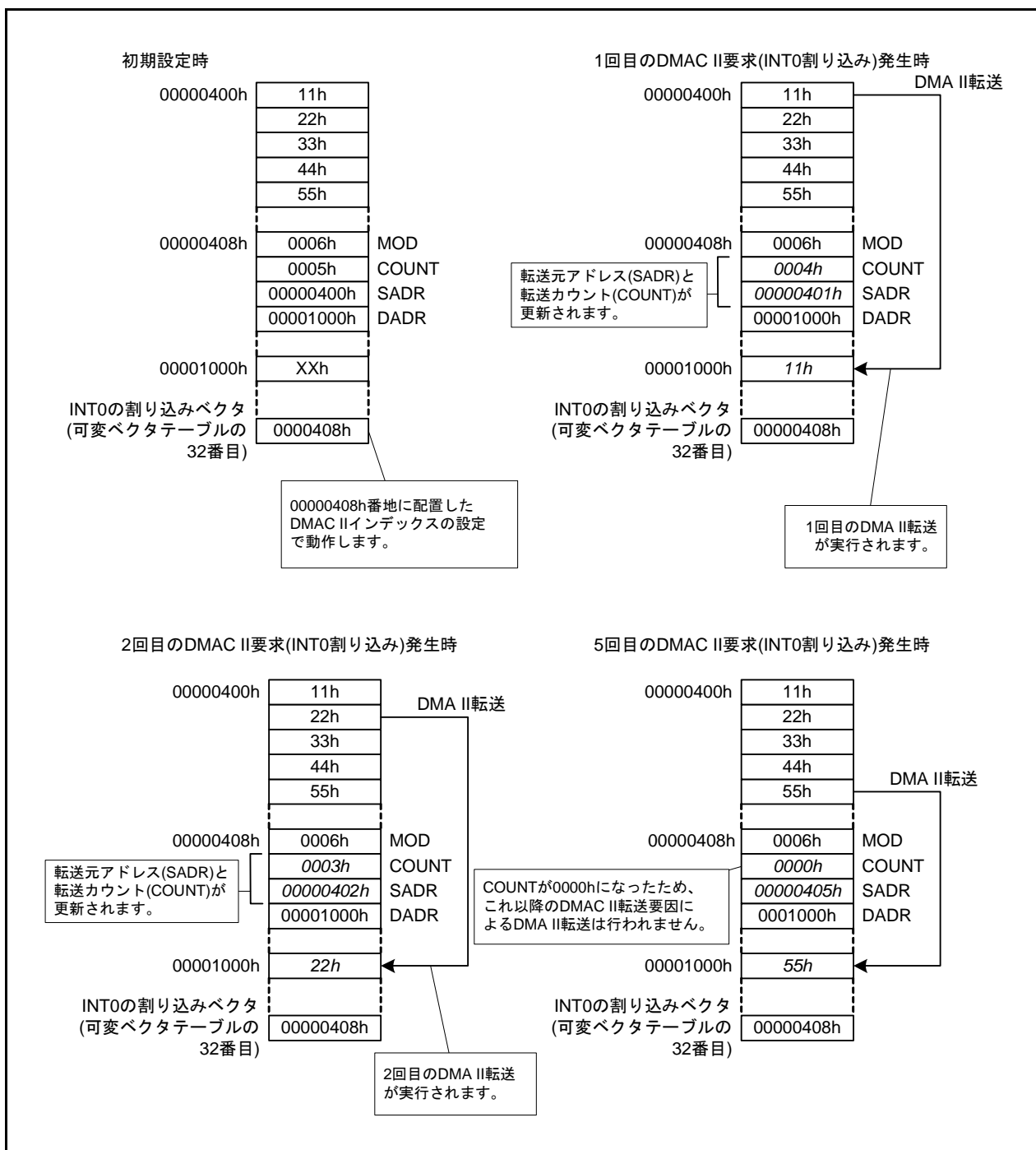
図 5.1 DMA II転送動作例
