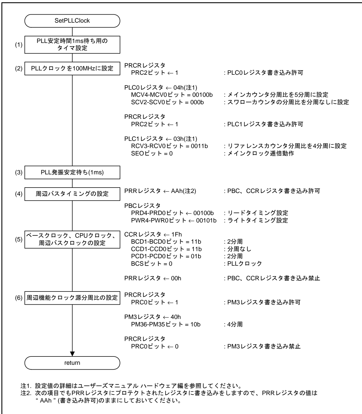
図 5.5 PLLクロック設定
