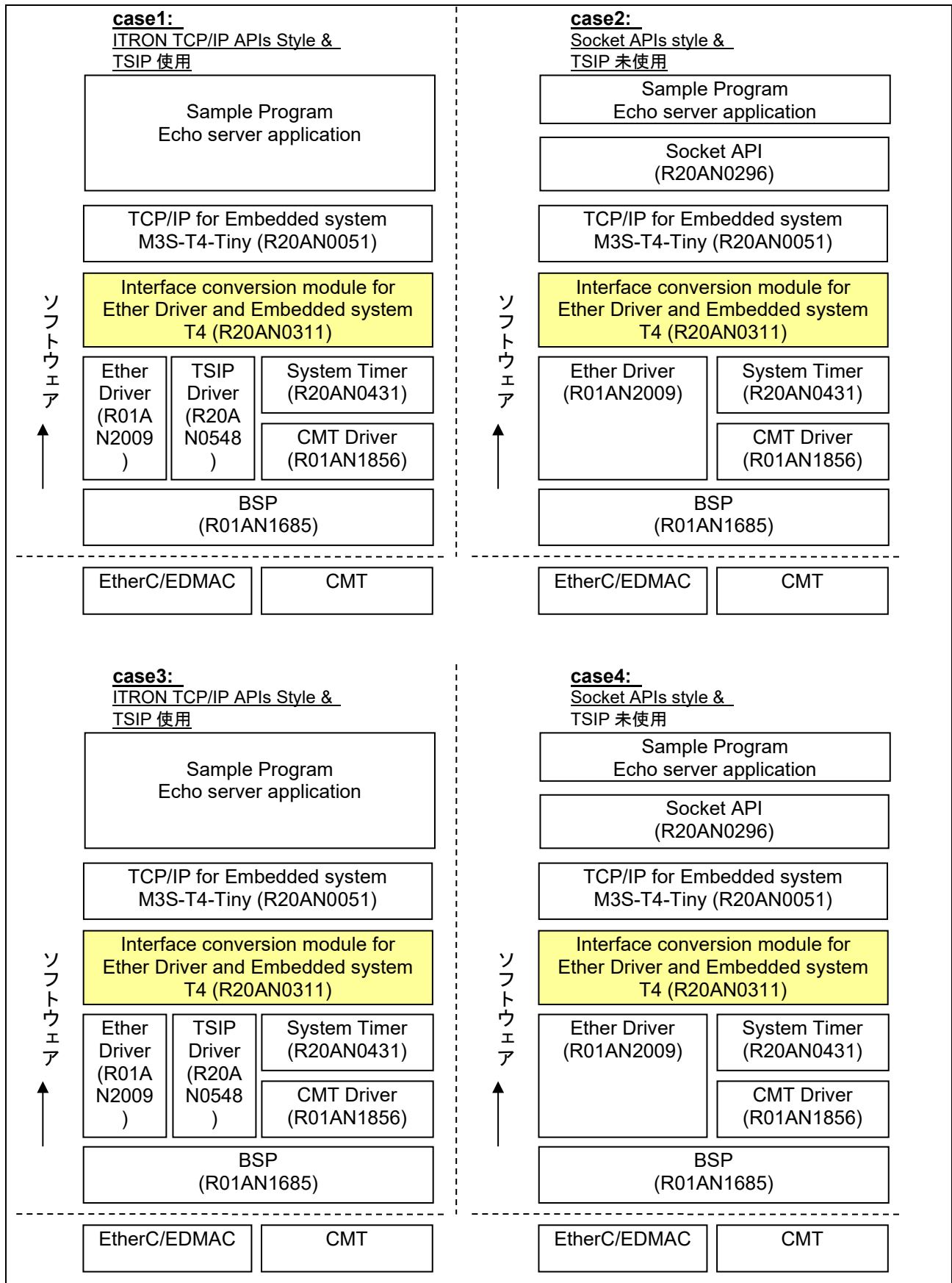
図 1 T4 ドライバ ソフトウェア構成
