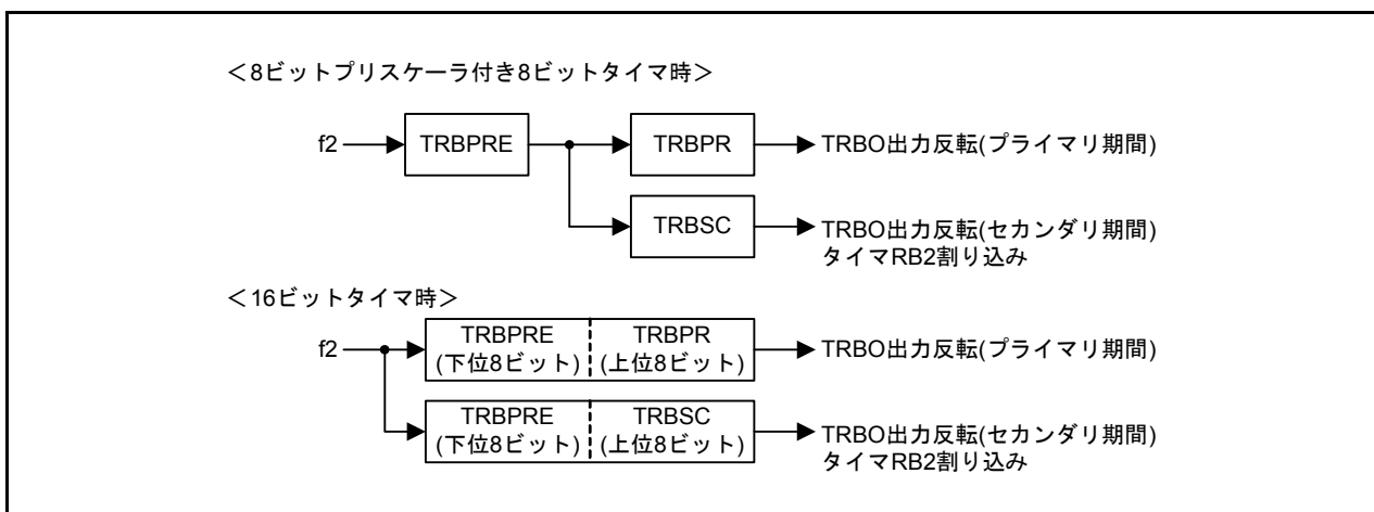
図 3.1 ブロック図
