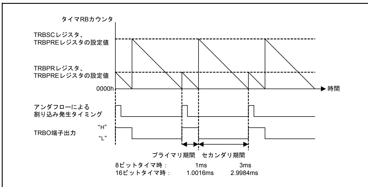
図 3.2 タイミング図
