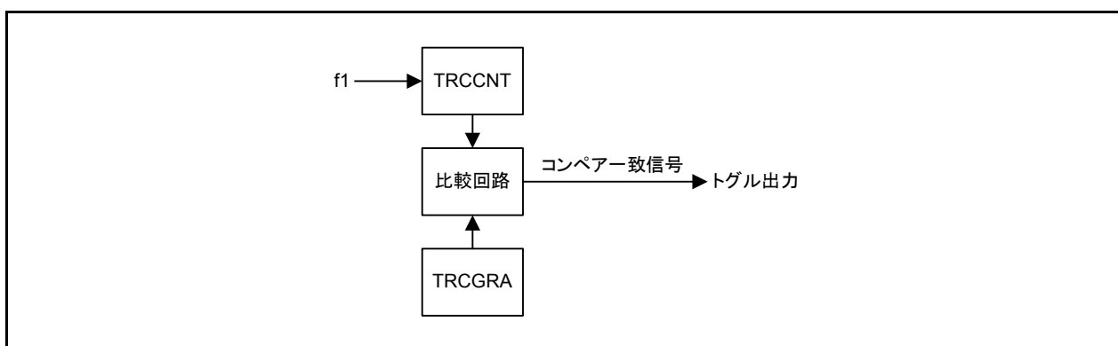
図 3.1 ブロック図
