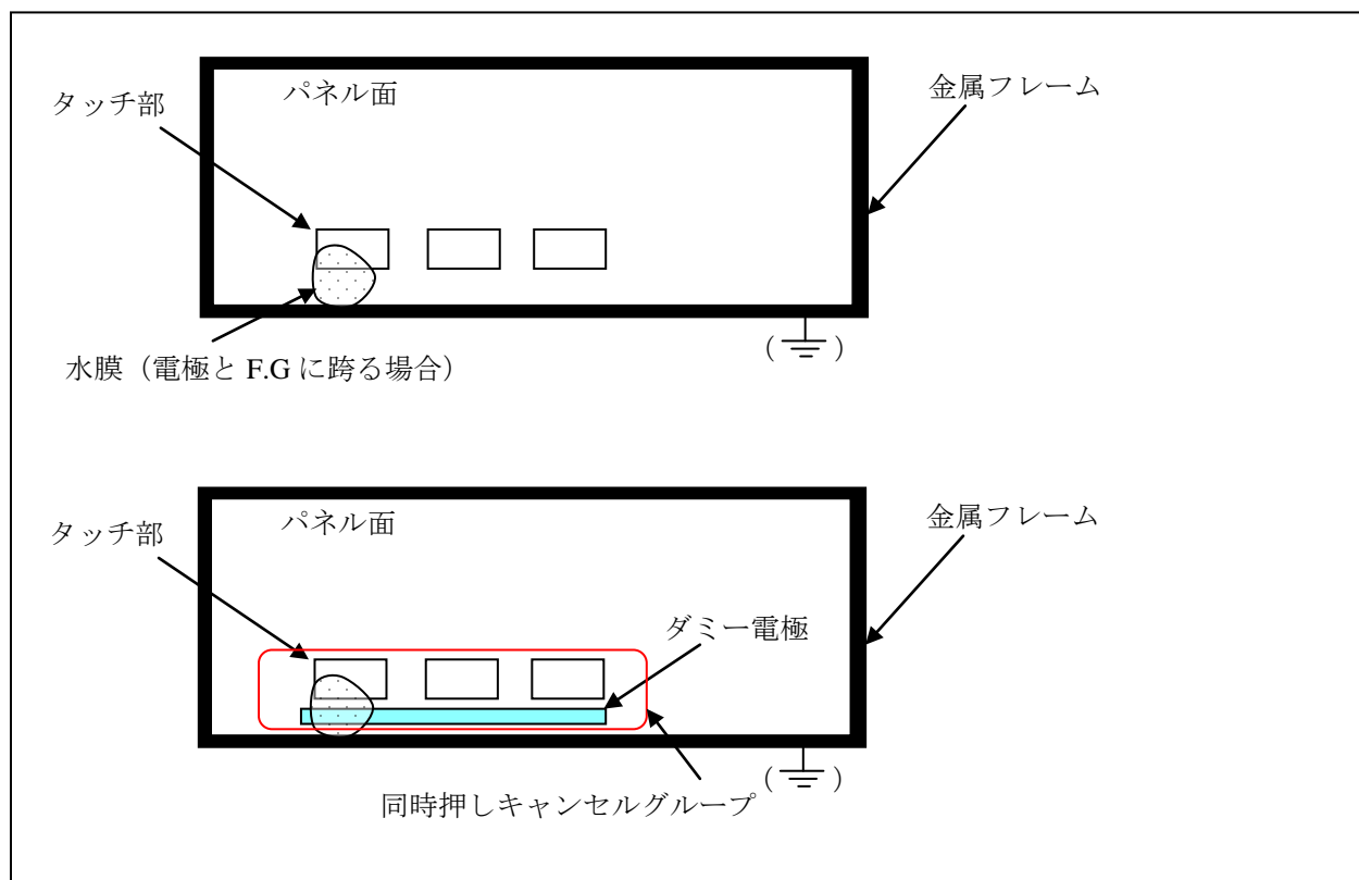
図 2-2-1 電極—GND間の水膜による影響の軽減方法
