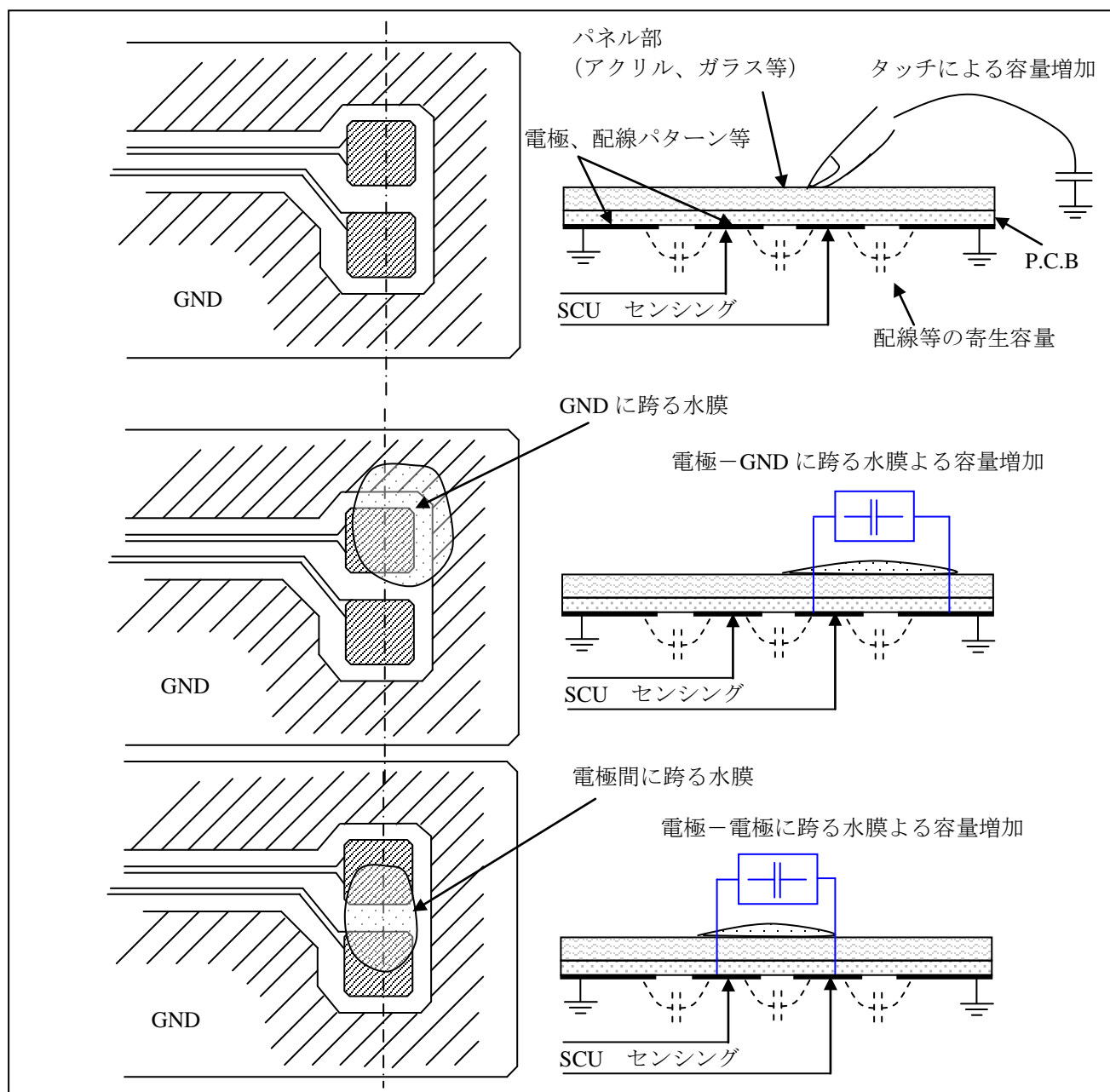
図 1-1-1 水膜によるタッチ誤判定
