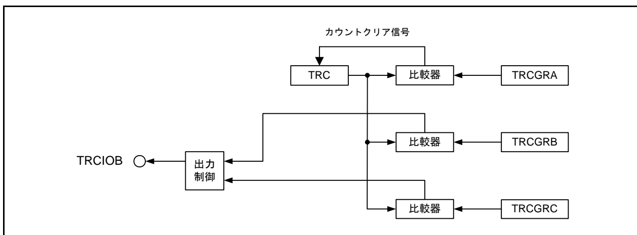
図 3.1 ブロック図
