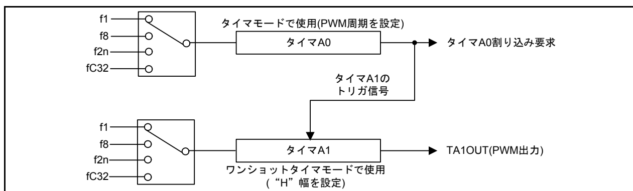
図 1.1 タイマ接続図
