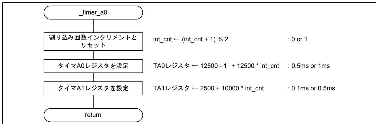
図 5.5 タイマA0割り込み処理
