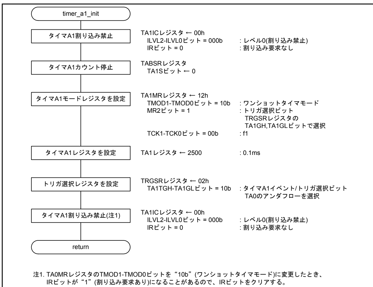
図 5.4 タイマA1初期設定処理
