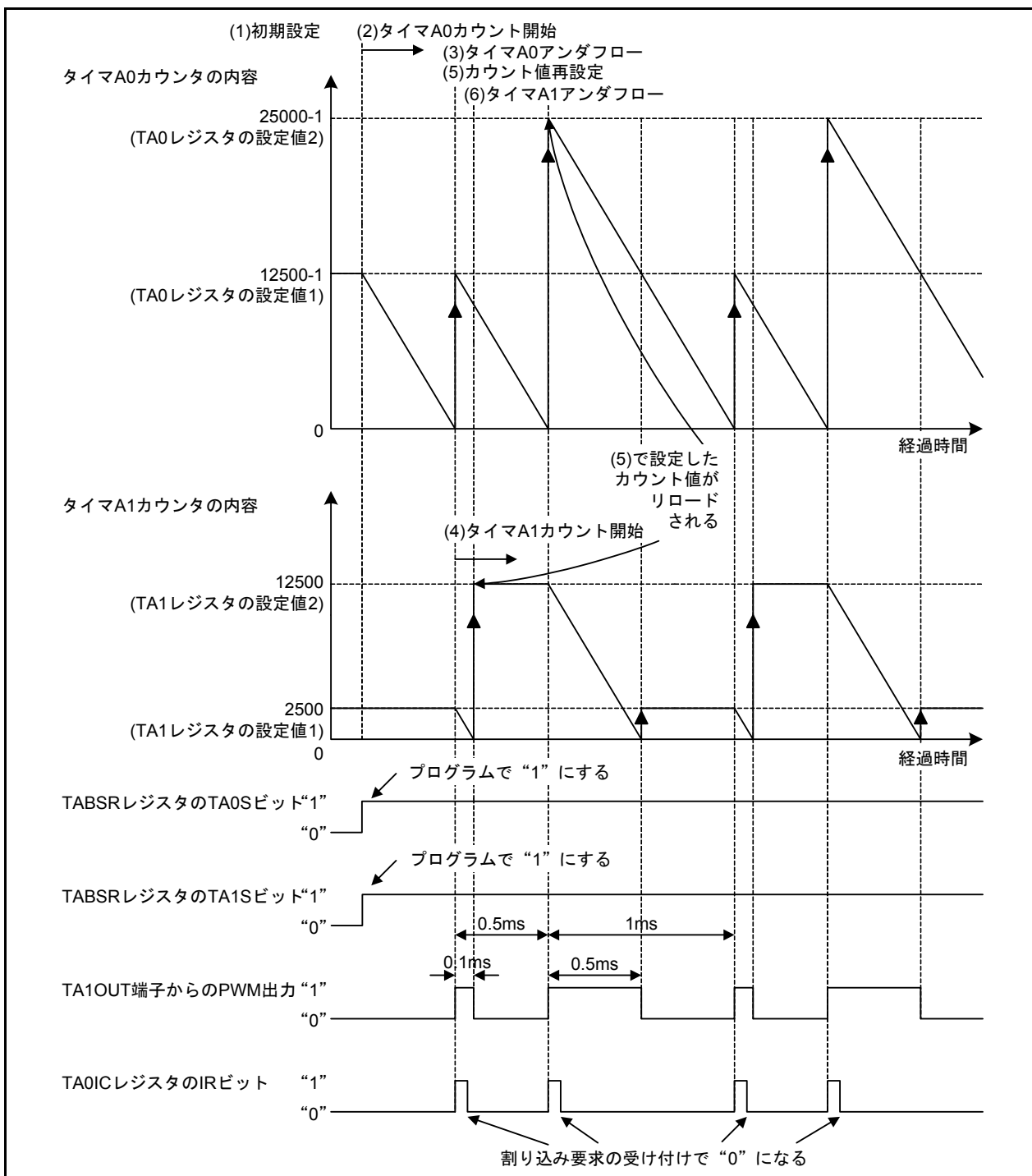
図 5.1 動作タイミング
