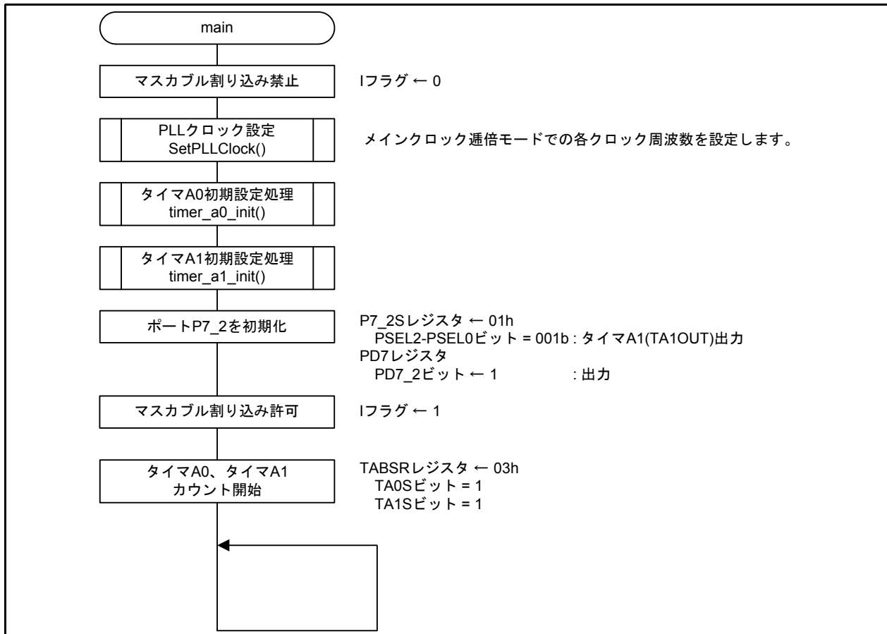
図 5.2 メイン処理
