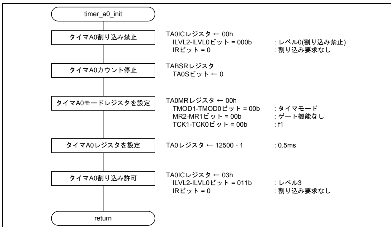
図 5.3 タイマA0初期設定処理
