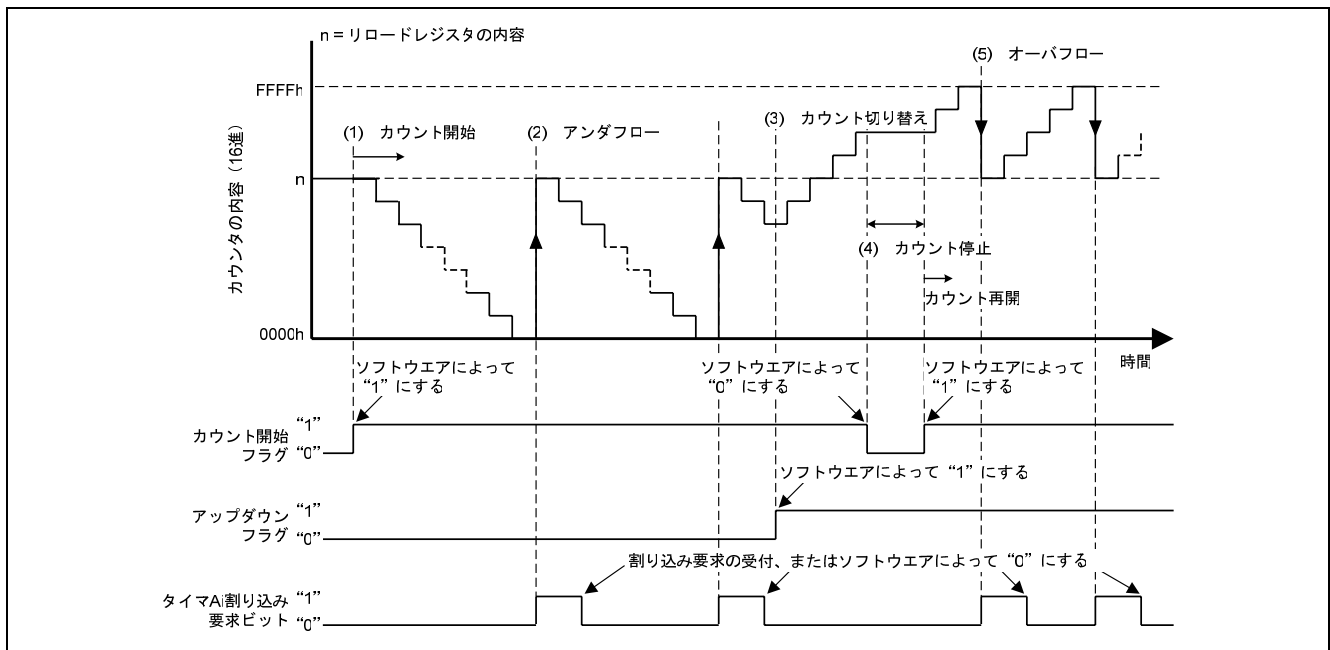
図 1. イベントカウンタモード、リロードタイプ選択時の動作タイミング
