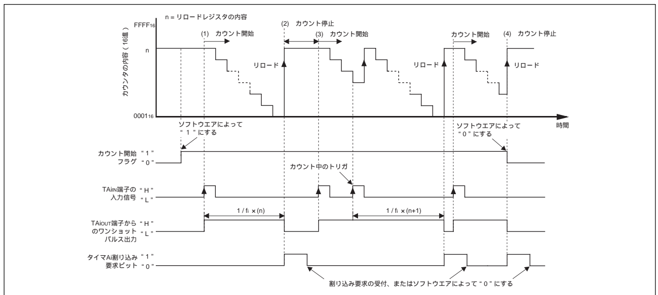
図1 ワンショットタイマモード、外部トリガ選択時の動作タイミング
