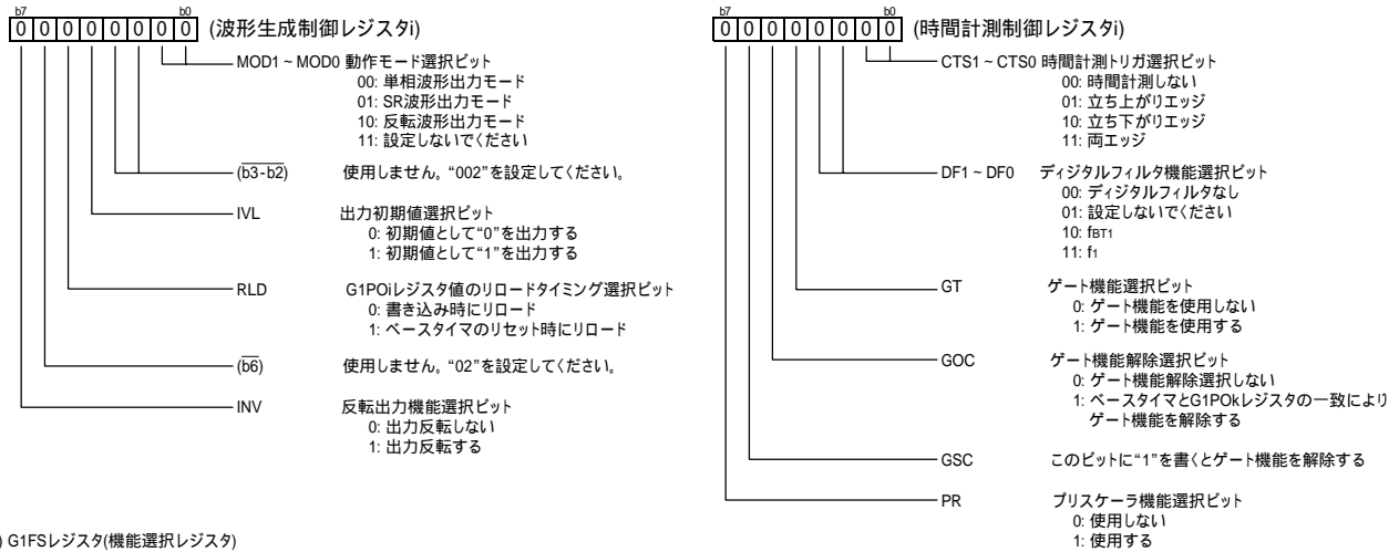
(2) G1FSレジスタ(機能選択レジスタ)
