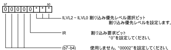
(5) ICOC0ICレジスタ(割り込み優先レベルの設定)
