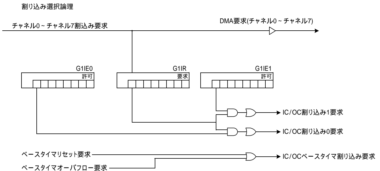
図 1IC/OC 割り込みと DMA 要求
