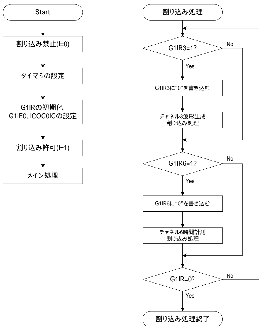
図 2 割り込み処理フロー
