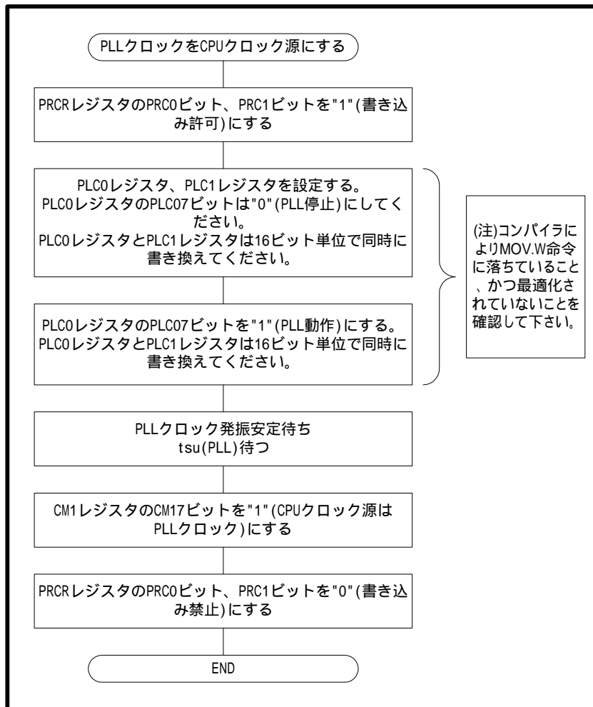
図 1 PLL クロックを CPU クロック源にするフロー図
