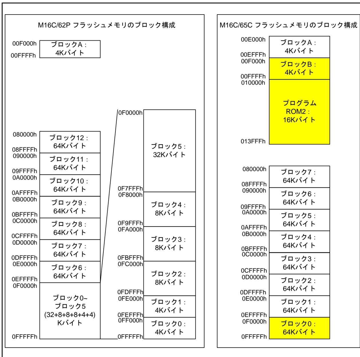
図 2.1 M16C/62PとM16C/65Cのフラッシュメモリのブロック構成の相違点
