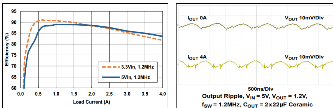
図 4: RAA210040 特性図 -- Vout=1.2V での効率 (左)、出力リップル (右)
