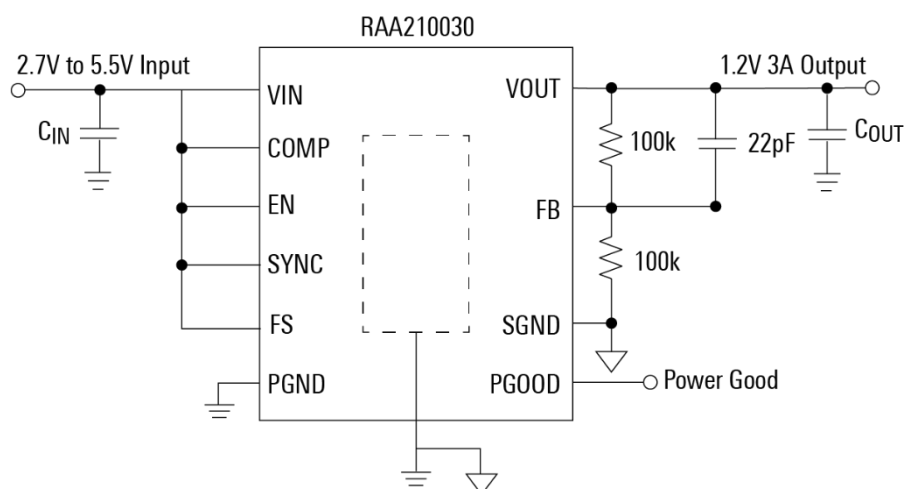
図 5 : RAA210030 の応用回路例
