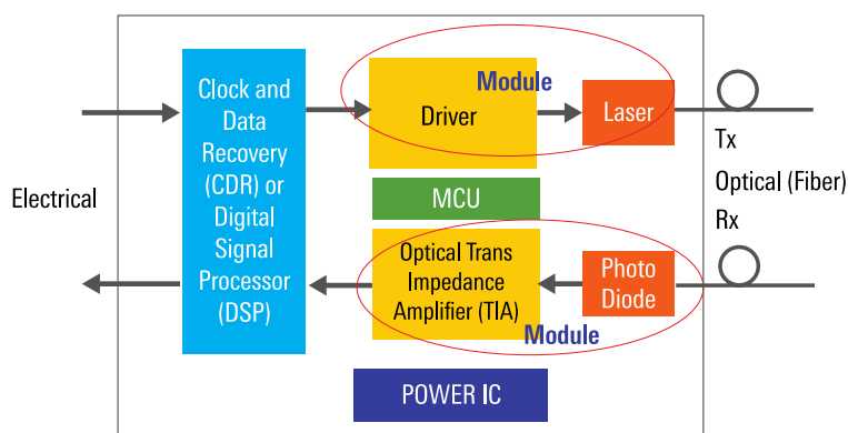
図 2: 光モジュール電力アーキテクチャ。赤い楕円はルネサスの小型電源モジュールの適用箇所を示しています。
