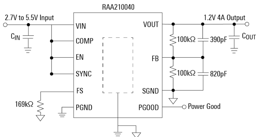
図 3: RAA210040 の応用回路例
