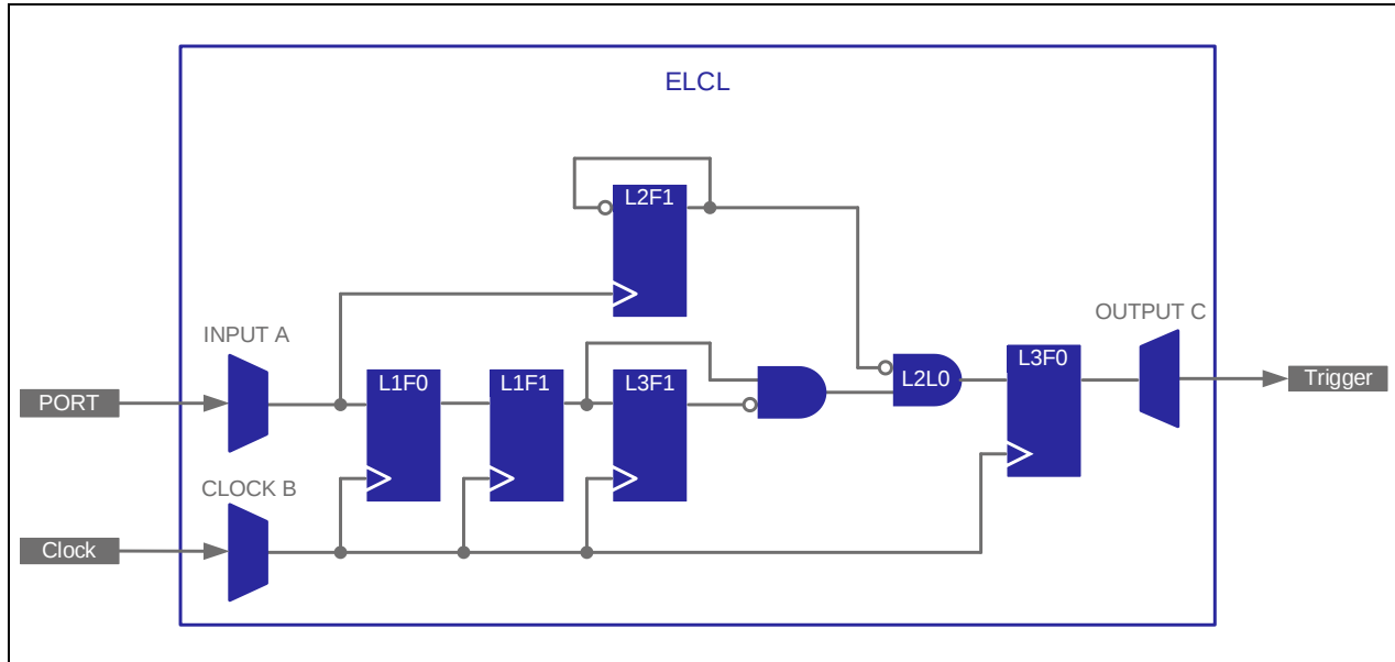
図 11：エッジ検出の間引きの構成
