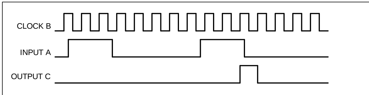
図 12：タイミングチャート
