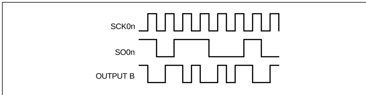
図 18 : タイミングチャート
