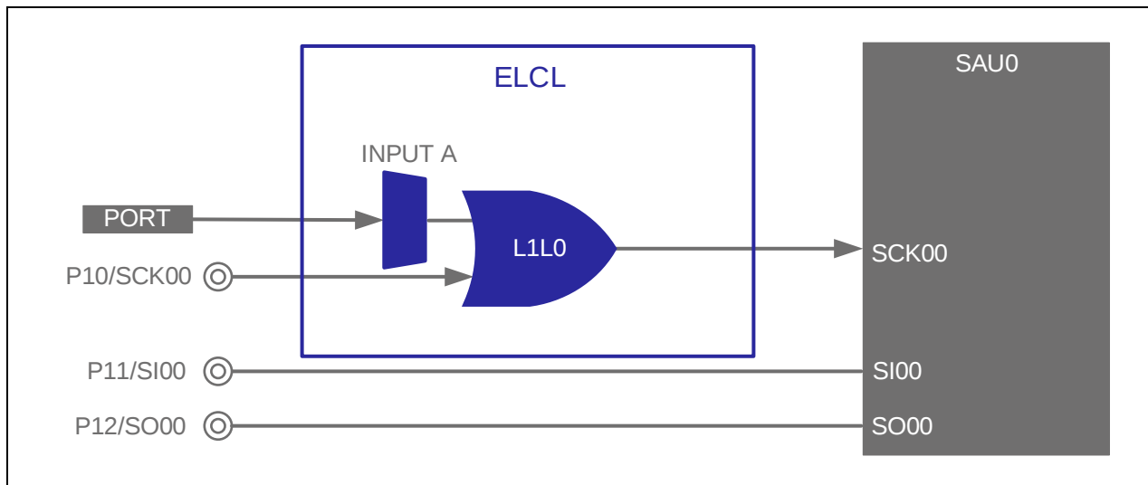
図 9：4 線式 SPI の構成
