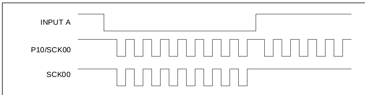
図 10：タイミングチャート
