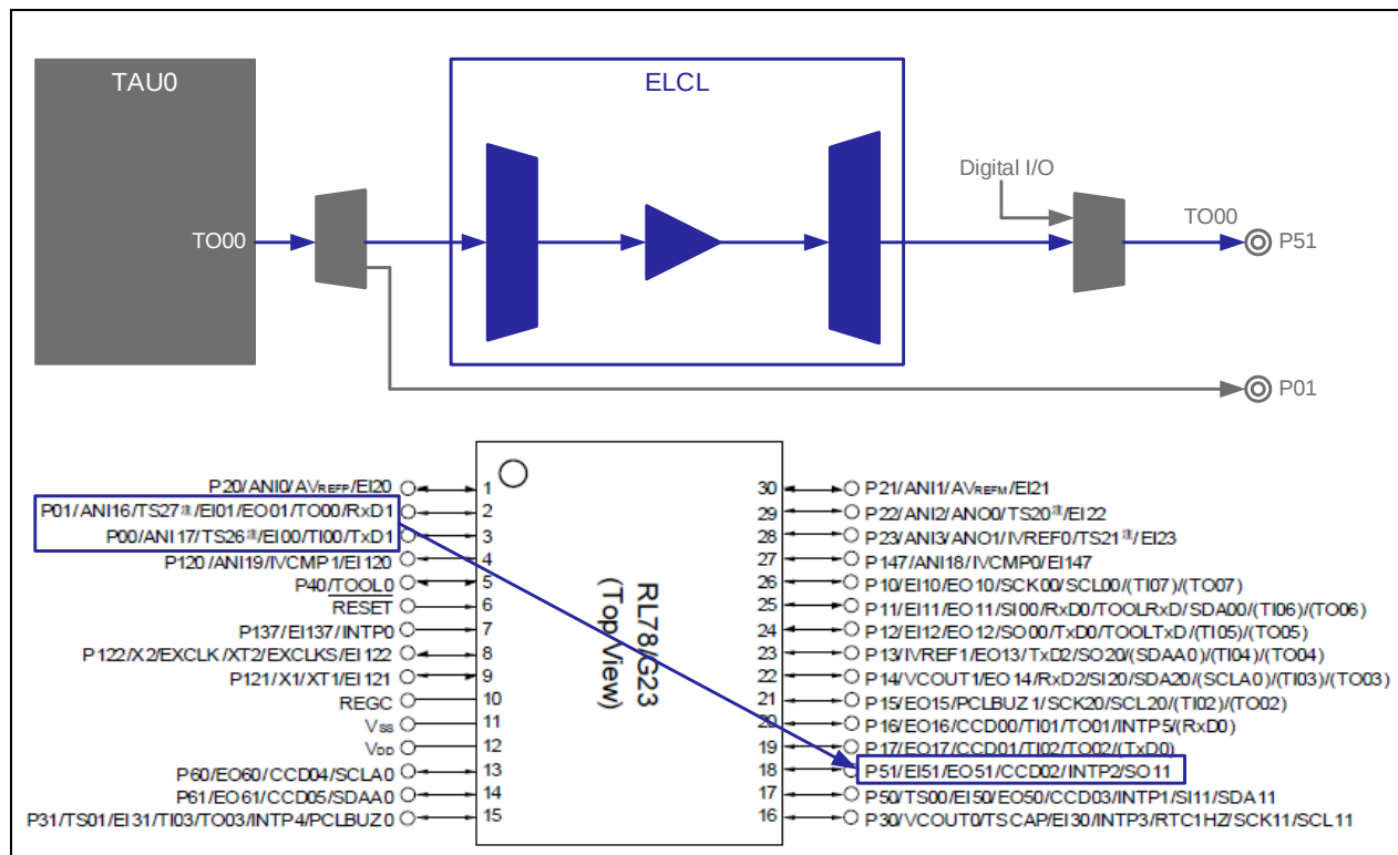
図 6：ELCL 機能例（出力端子の変更）
