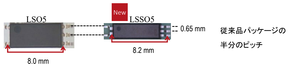
図 2. 従来の LSO5 パッケージと新 LSSO5 パッケージの比較
