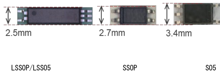
図 5. LSS05/LSS0P、SS0P、S05 パッケージの比較
