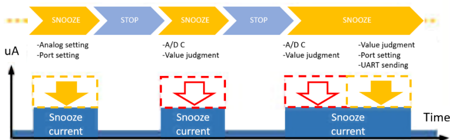
図 4：RL78/G23 のインテリジェント・スヌーズ機能
