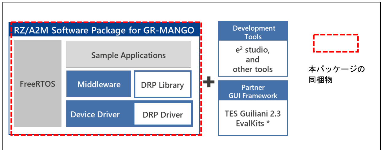
図 1 RZ/A2M Software Package for GR-MANGO の構成イメージ
