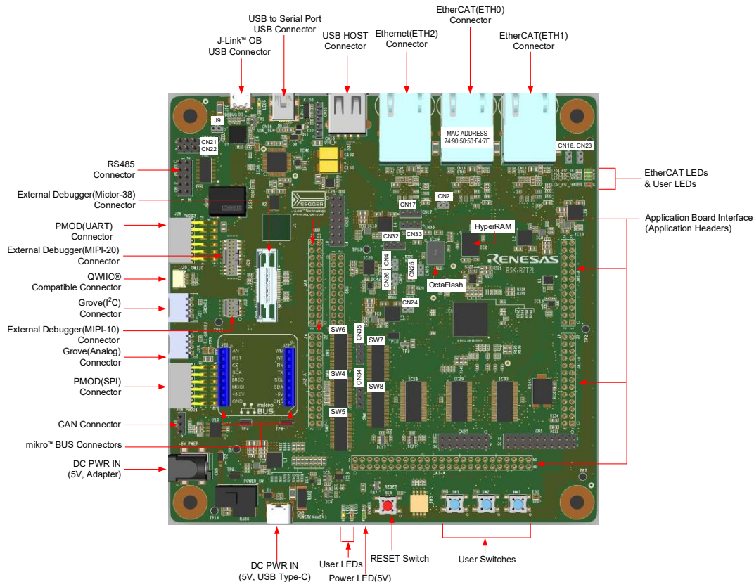
図 2 CPU ボード図 (部品面)
