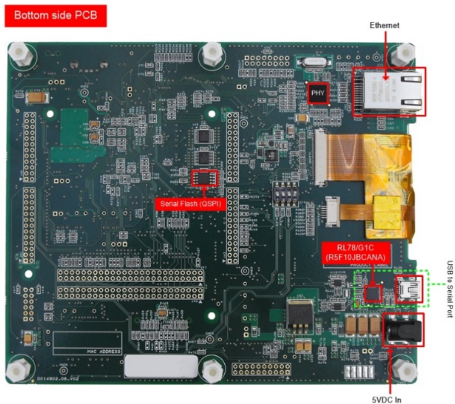
図3 CPUボードの裏面図
