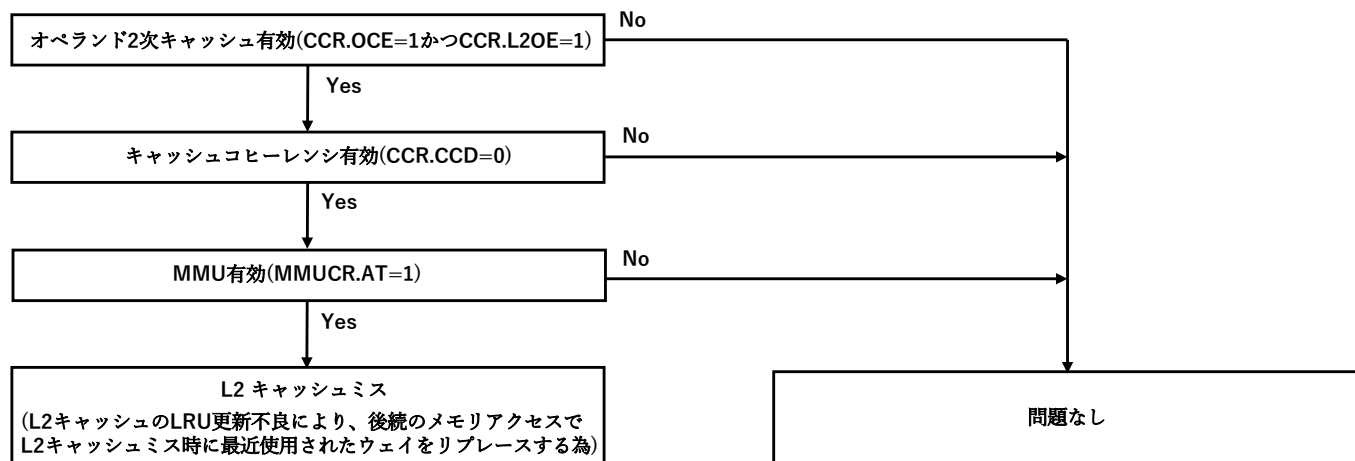
図 A.15 L2 キャッシュミスの発生条件
