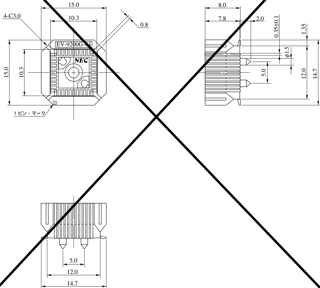
図A - 2 EV-9200G-44 外形図 (参考) (単位 : mm)
