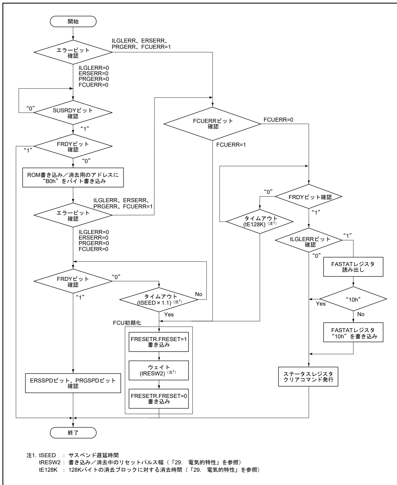
図 26.19 書き込み/消去のサスペンド方法
