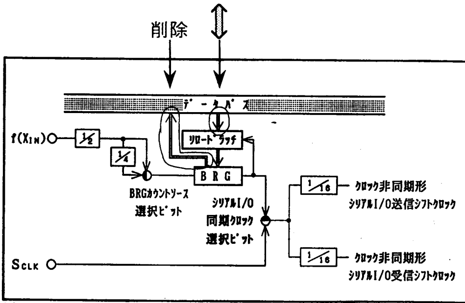
図2.7.9 ボーレートジェネレータ構成図 (2-71ページ)
