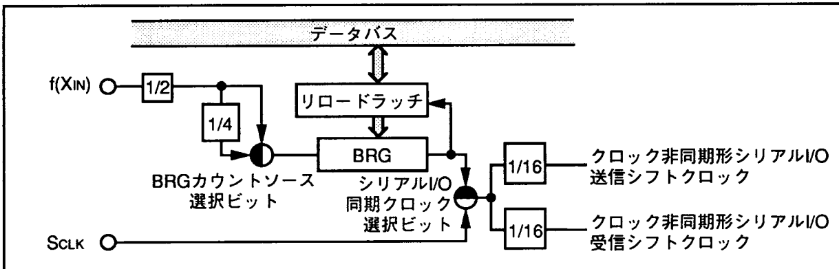
図2.7.9 クロック非同期形のボーレートジェネレータ構成
