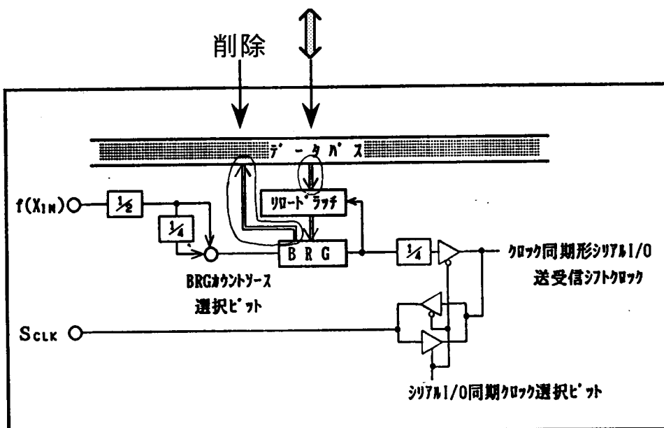
図2.7.2 ボーレートジェネレータ構成図 (2-58ページ)
