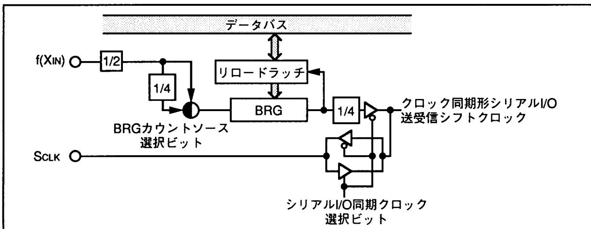
図2.7.2 クロック同期形のボーレートジェネレータ構成
