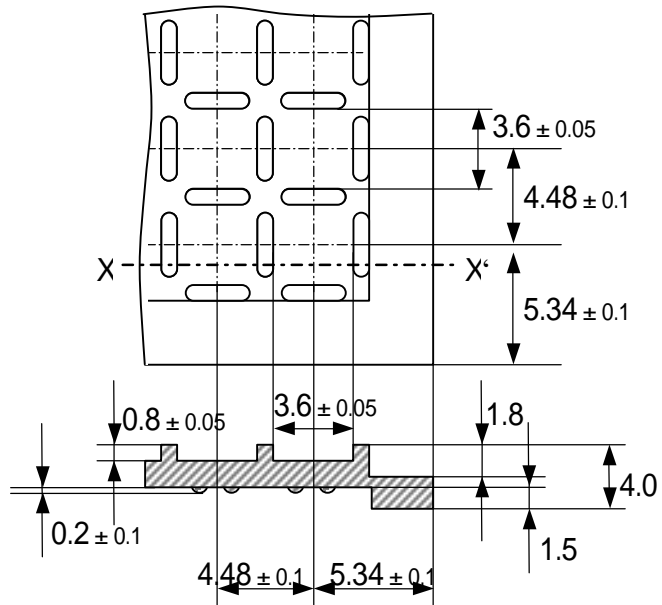
X-X' 断面図
