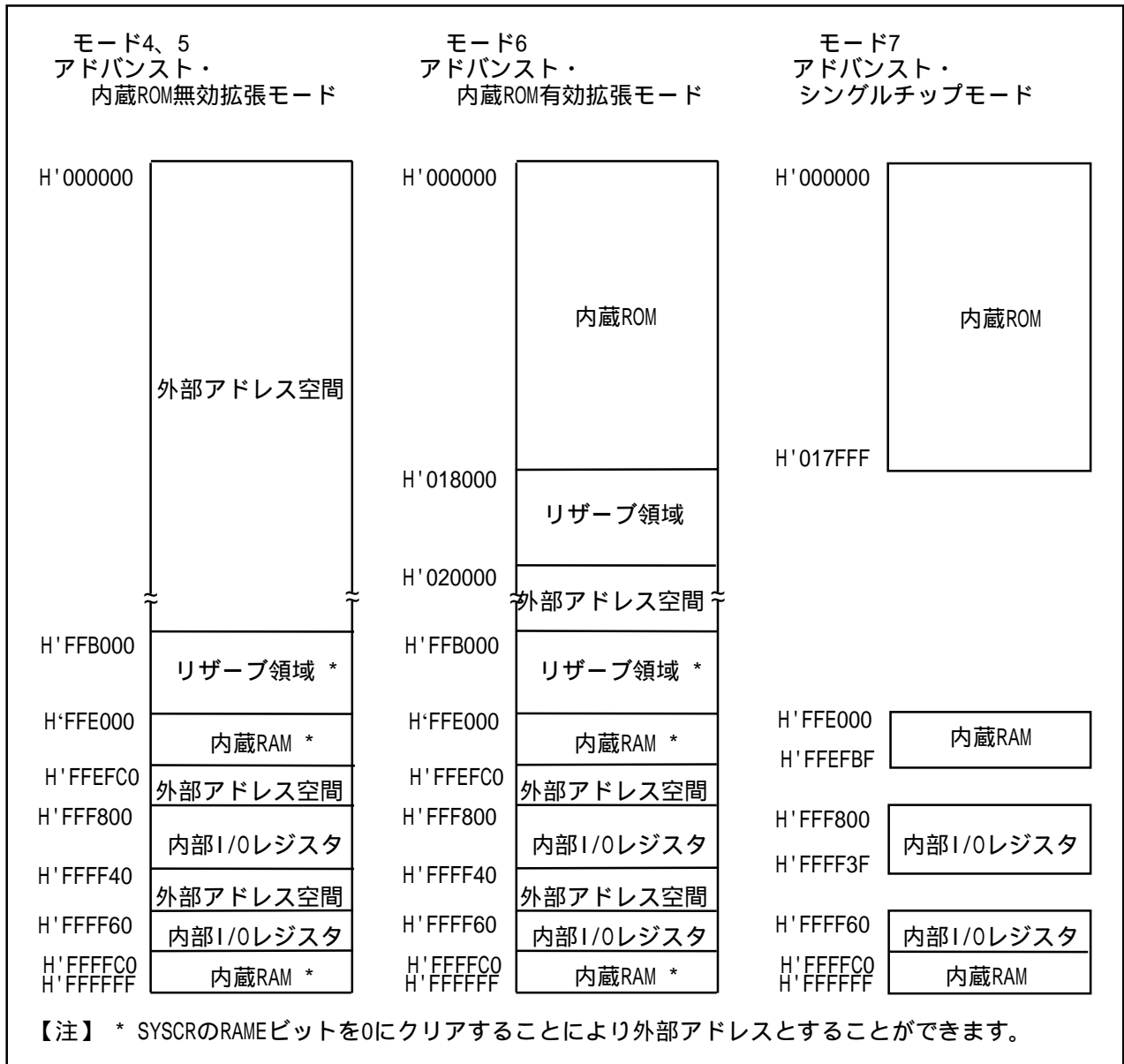
図3.3 H8S/2224の各動作モードのアドレスマップ
