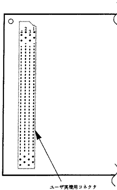
図3.6 H8/500シリーズ小型エバボード実装図
