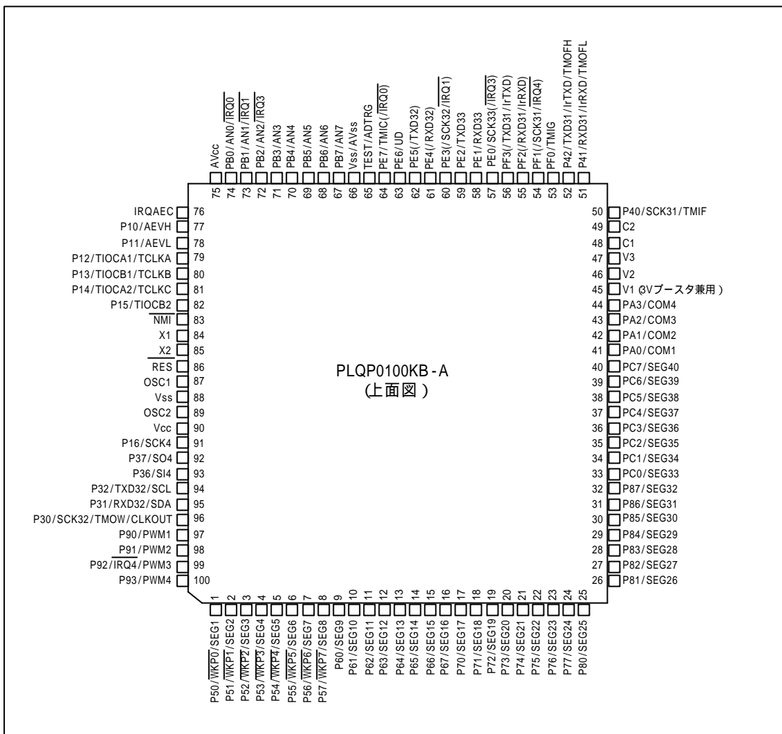
図1.2 H8/38099 グループピン配置図 (PLQP0100KB - A)
