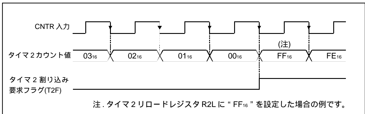
図. タイマ2カウンタ動作タイミング (カウンタソースに CNTR 入力選択時)
