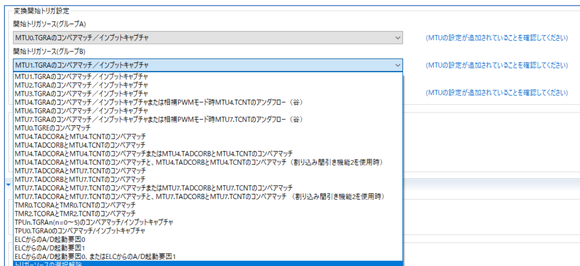
図 3-2 開始トリガソース(グループ B)の選択肢
