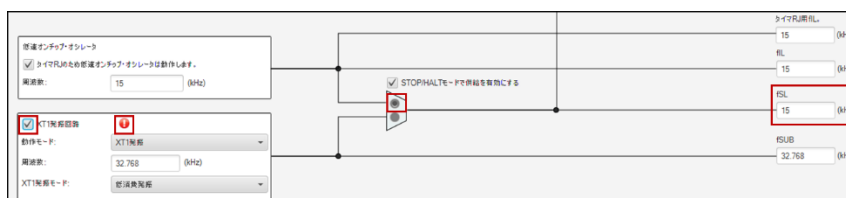
図 3-1 低速オンチップ・オシレータ動作時、XT1 発振回路は使用不可
