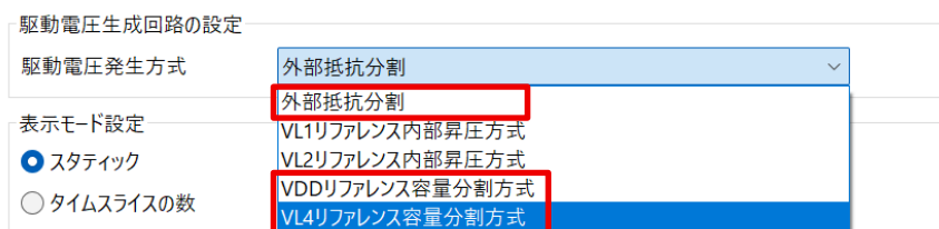
図 5-7 駆動電圧発生方式
