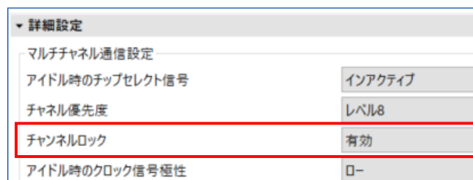
図 3-2 MSPI マスタチャネル ロック設定
