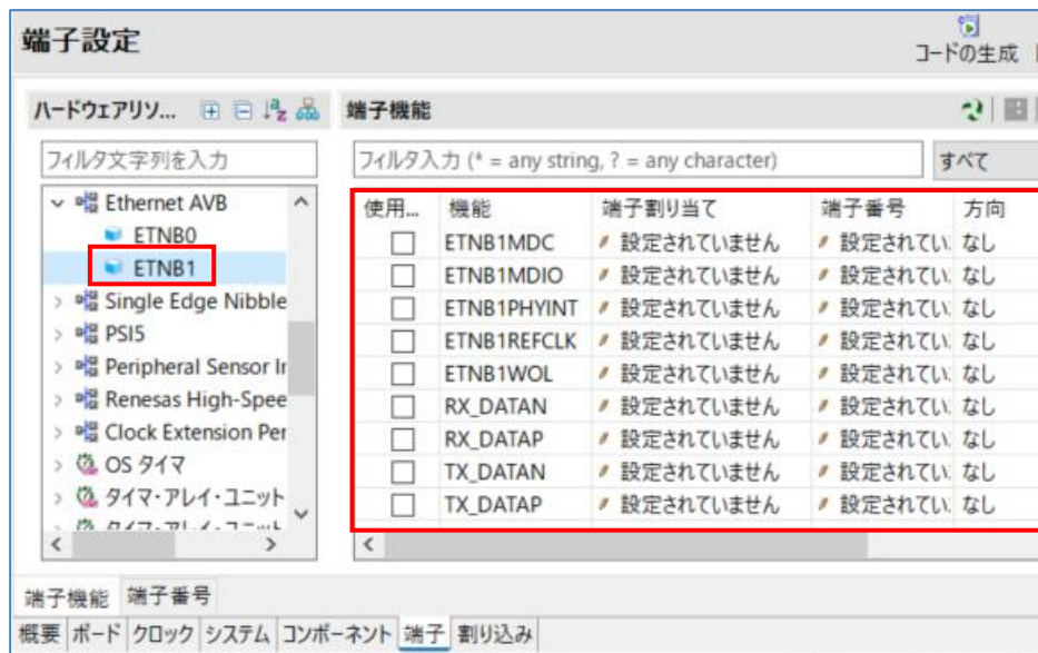
図 3-6 ETNB1 の端子設定
