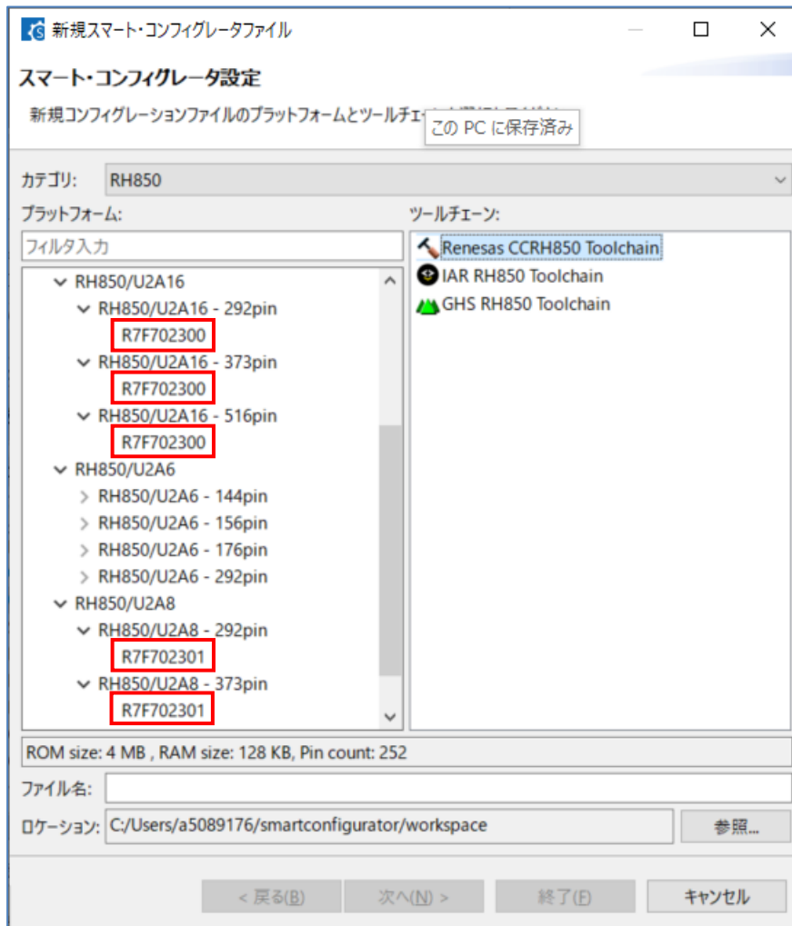
図 3-7 U2A のデバイス表示
