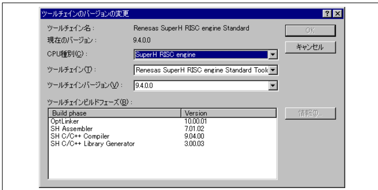
図 3.4 [ツールチェーンのバージョンの変更]ダイアログボックス
