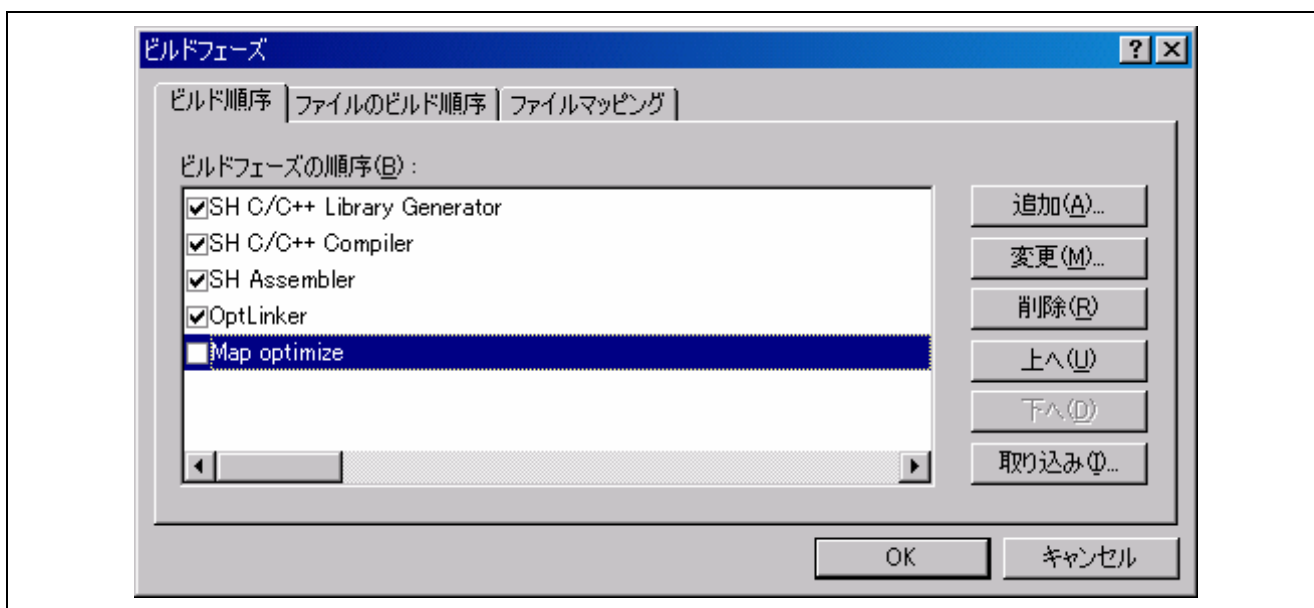
図 3.1 [ビルドフェーズ]ダイアログボックス
