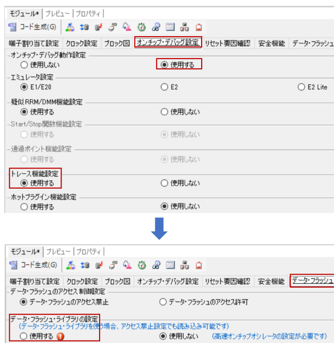
図 6-6 トレース機能とデータ・フラッシュ・ライブラリを併用できない場合
