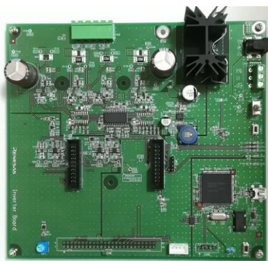
(1)インバータボード
