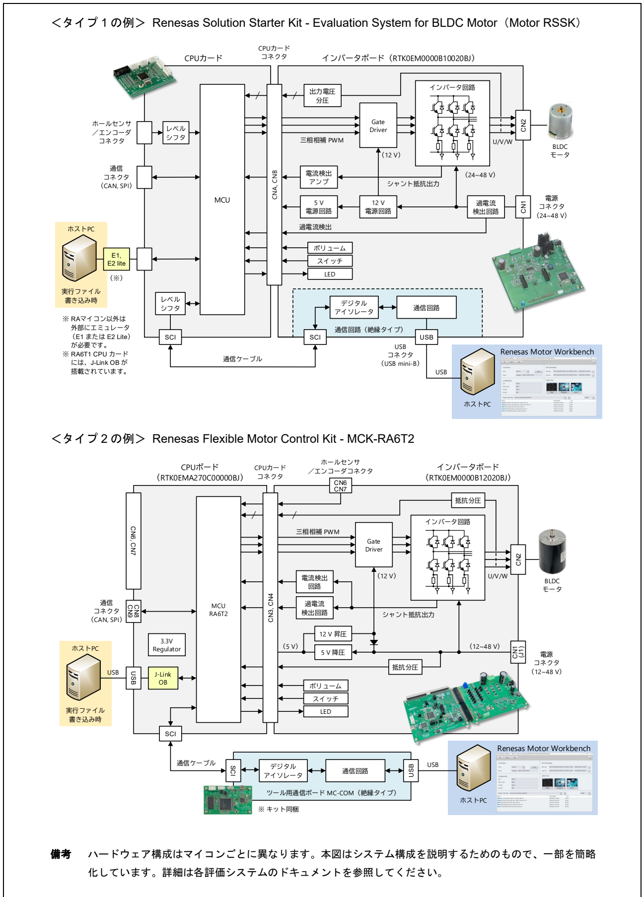
図 1-3 ルネサスモータ評価システムのハードウェア構成図 (図 1-2 のタイプ 1 とタイプ 2 の例)
