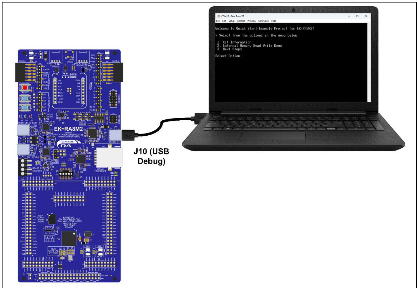
図 3. EK-RA8M2 ボードを USB デバッグ経由でホスト PC に接続
