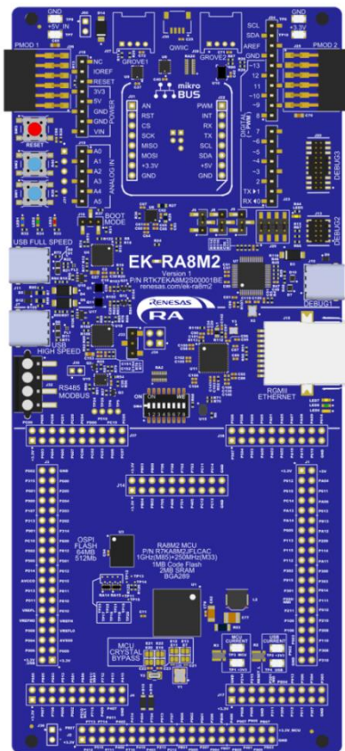
図 1. EK-RA8M2 キットの構成
