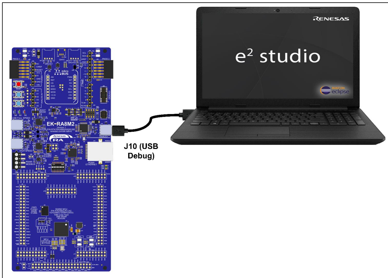
図 25. USB デバッグポートを使用した EK-RA8M2 ボードとホスト PC の接続
