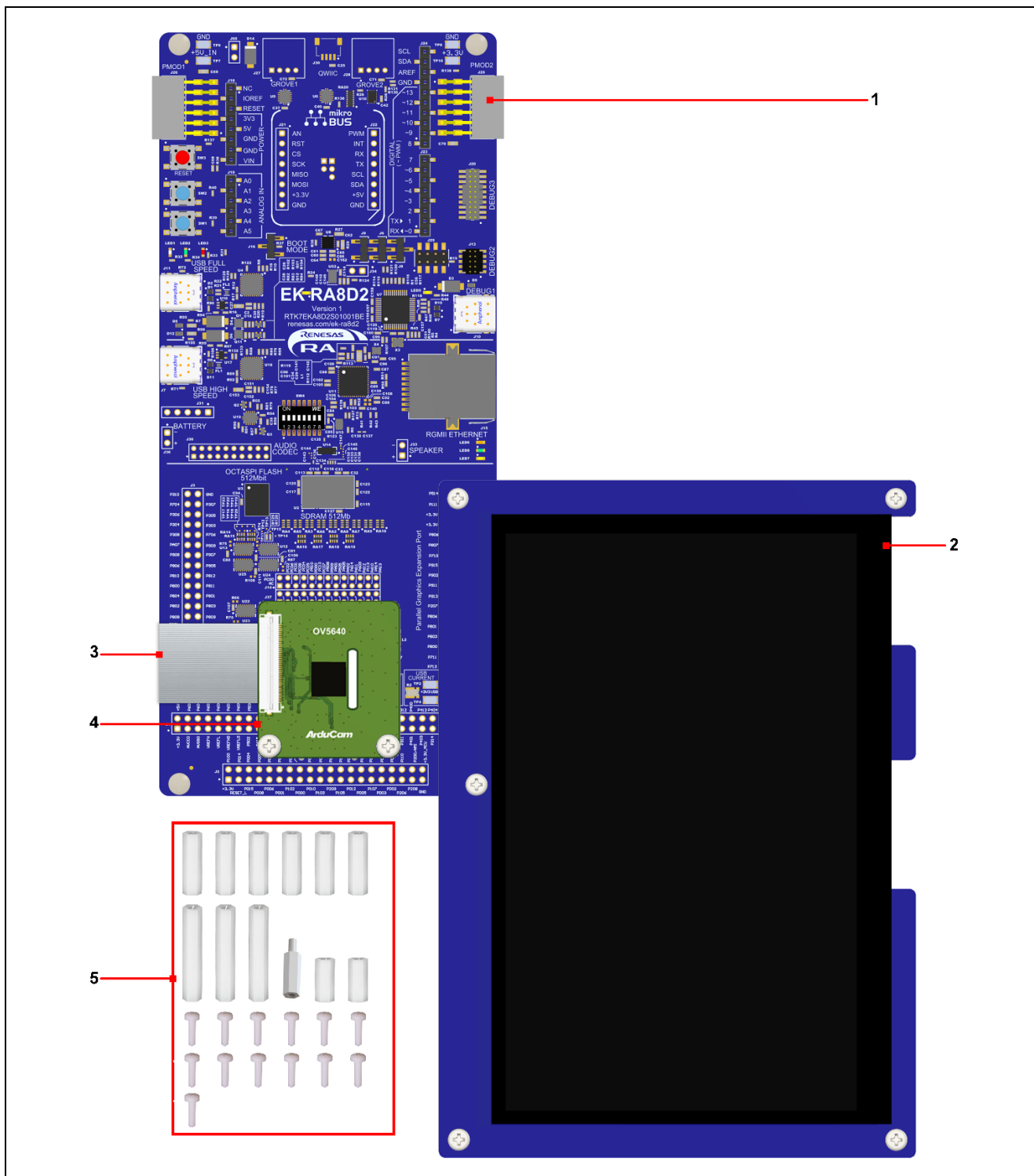
図 1. EK-RA8D2 キットの構成
