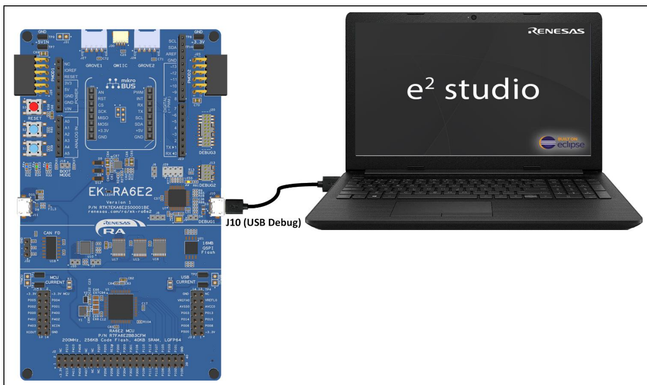
図 23. USB デバッグポートを使用した EK-RA6E2 ボードとホスト PC の接続
