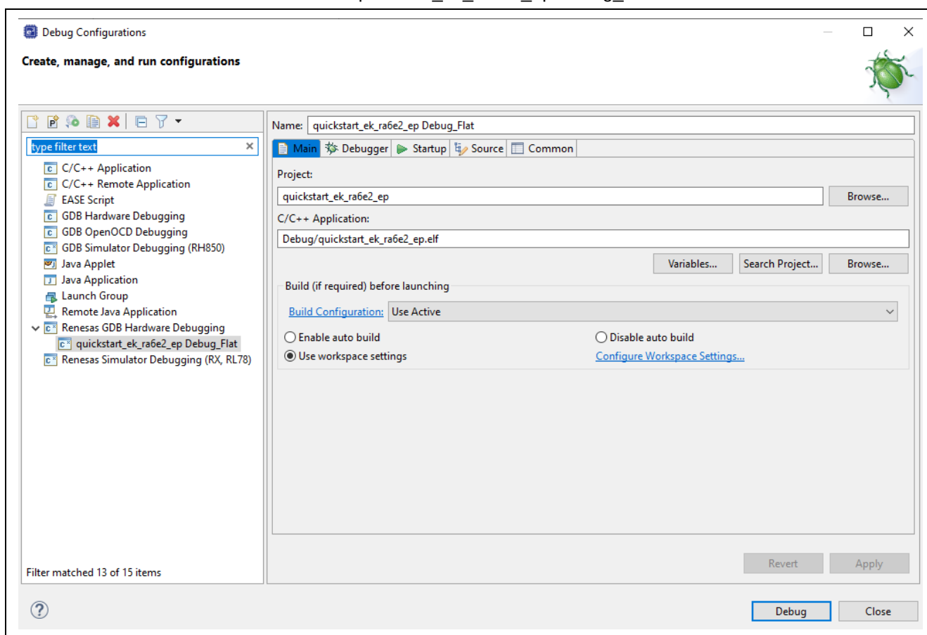
図 25. デバッグイメージの選択
