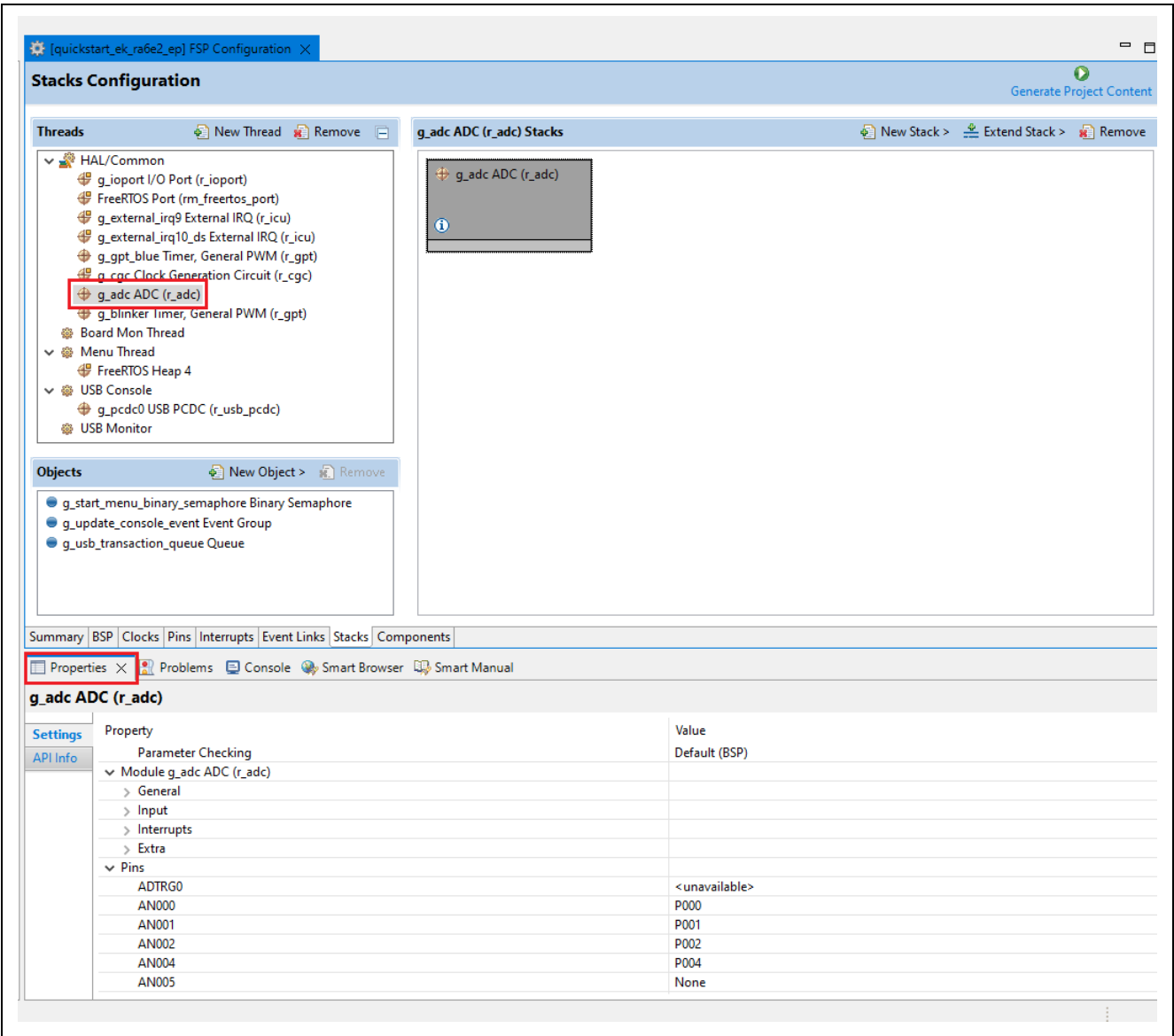
図 19. 構成設定の変更
