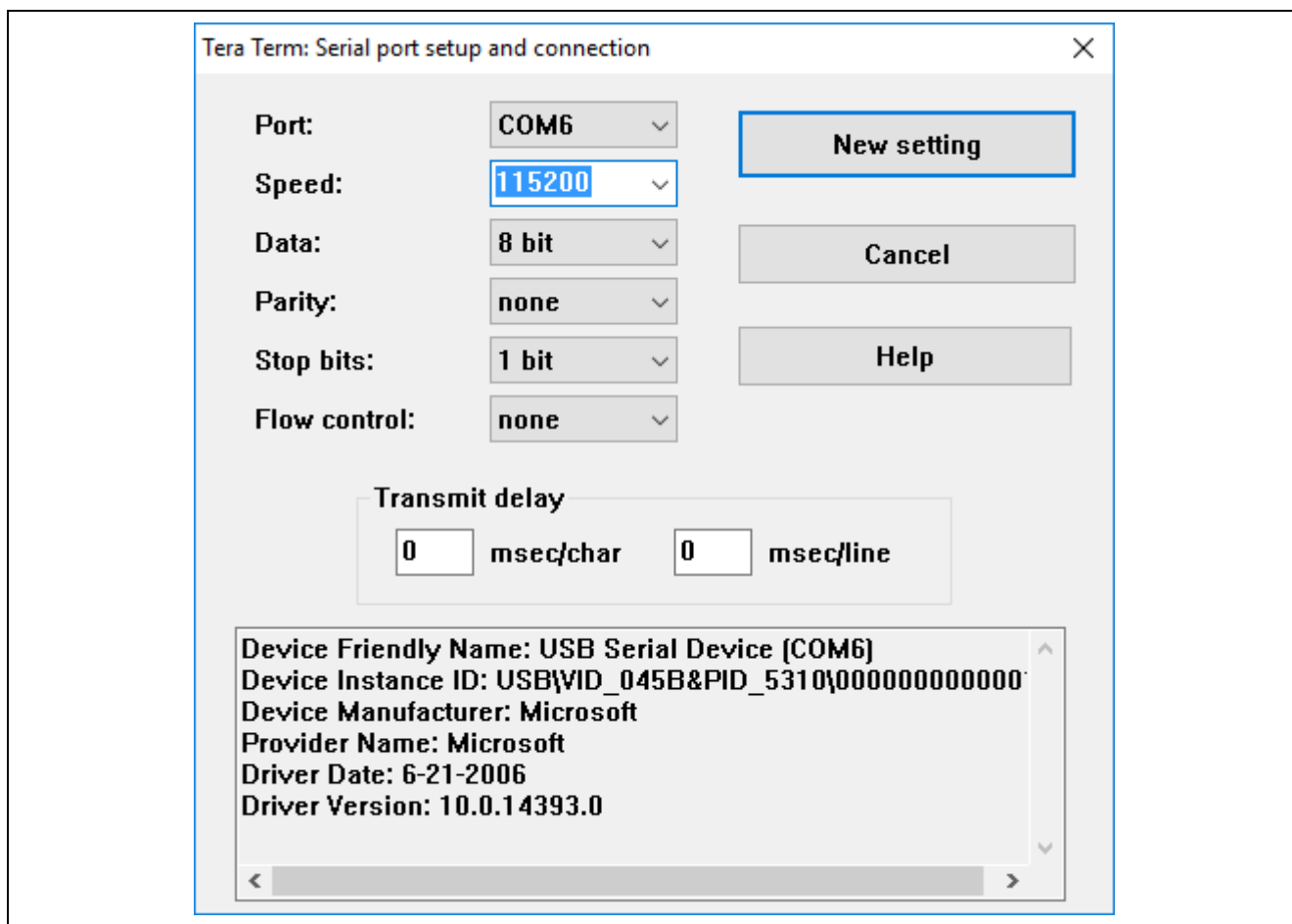
図 6. スピードプルダウンで 115200 を選択
