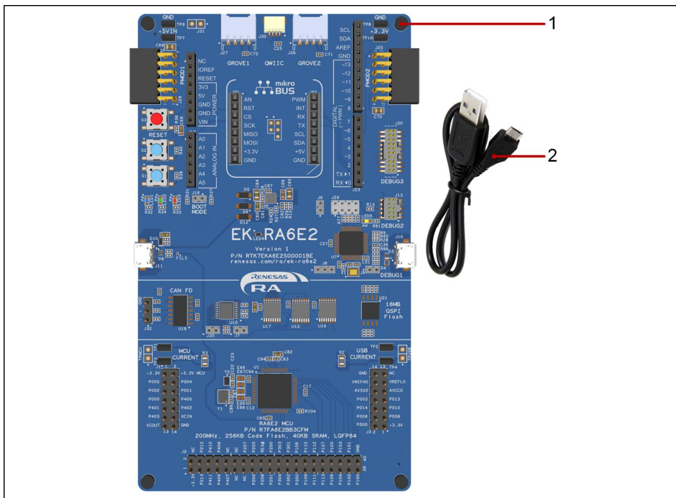
図 1. EK-RA6E2 評価キット構成
