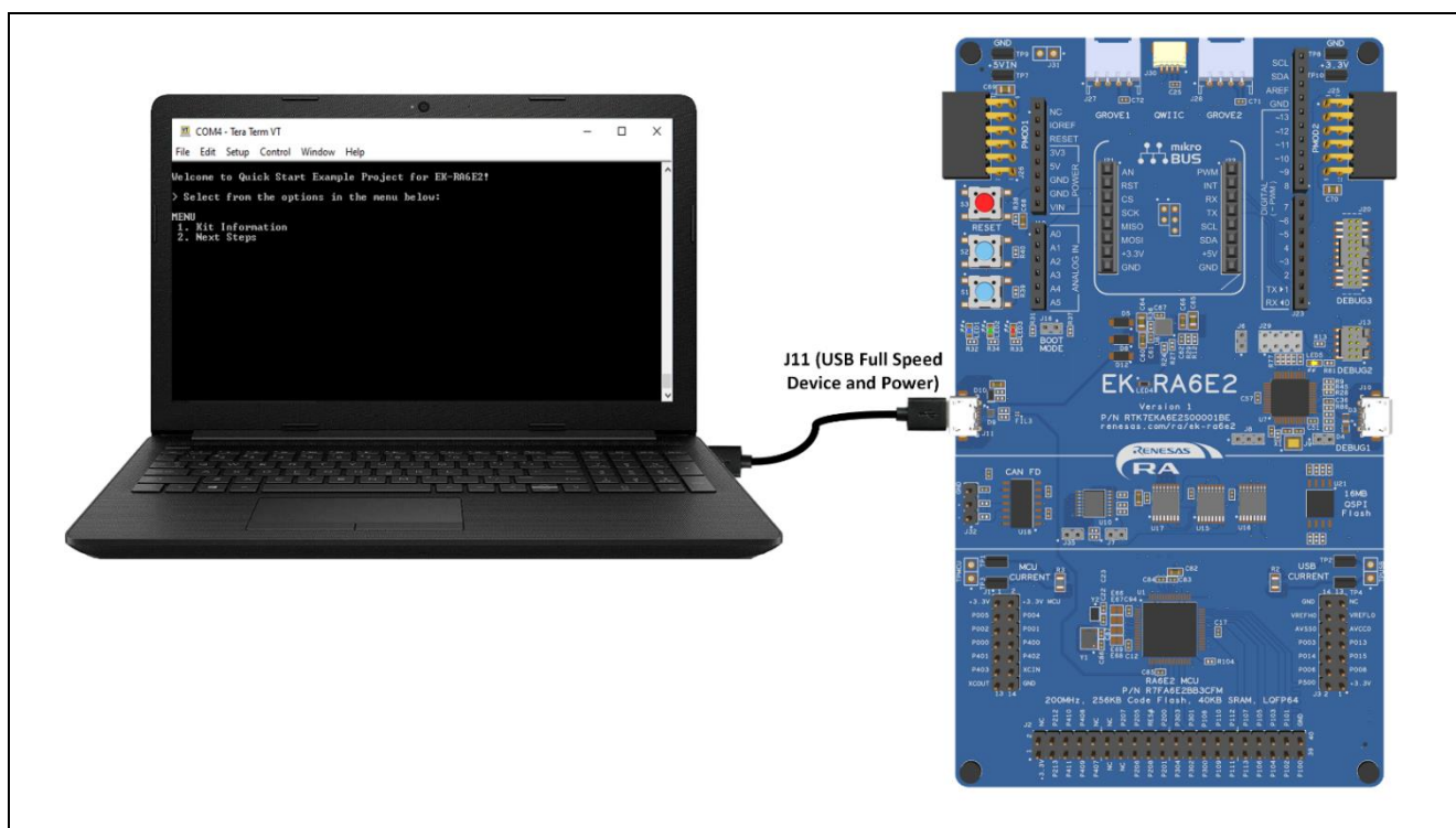
図 3. EK-RA6E2 ボードを USB フルスピード ポート経由でホスト PC に接続
