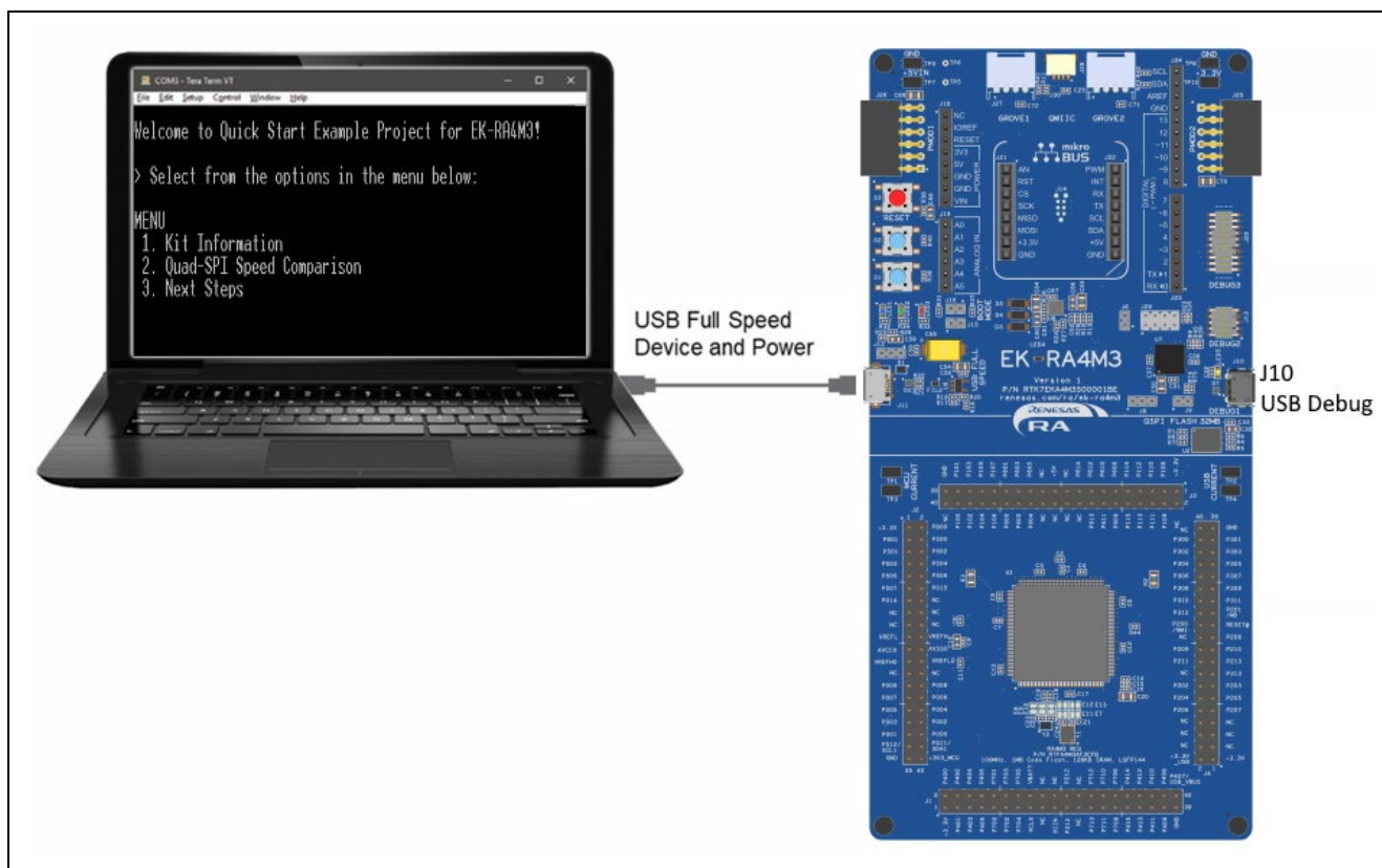
図 3 USB フルスピードポートでボードをホスト PC に接続
