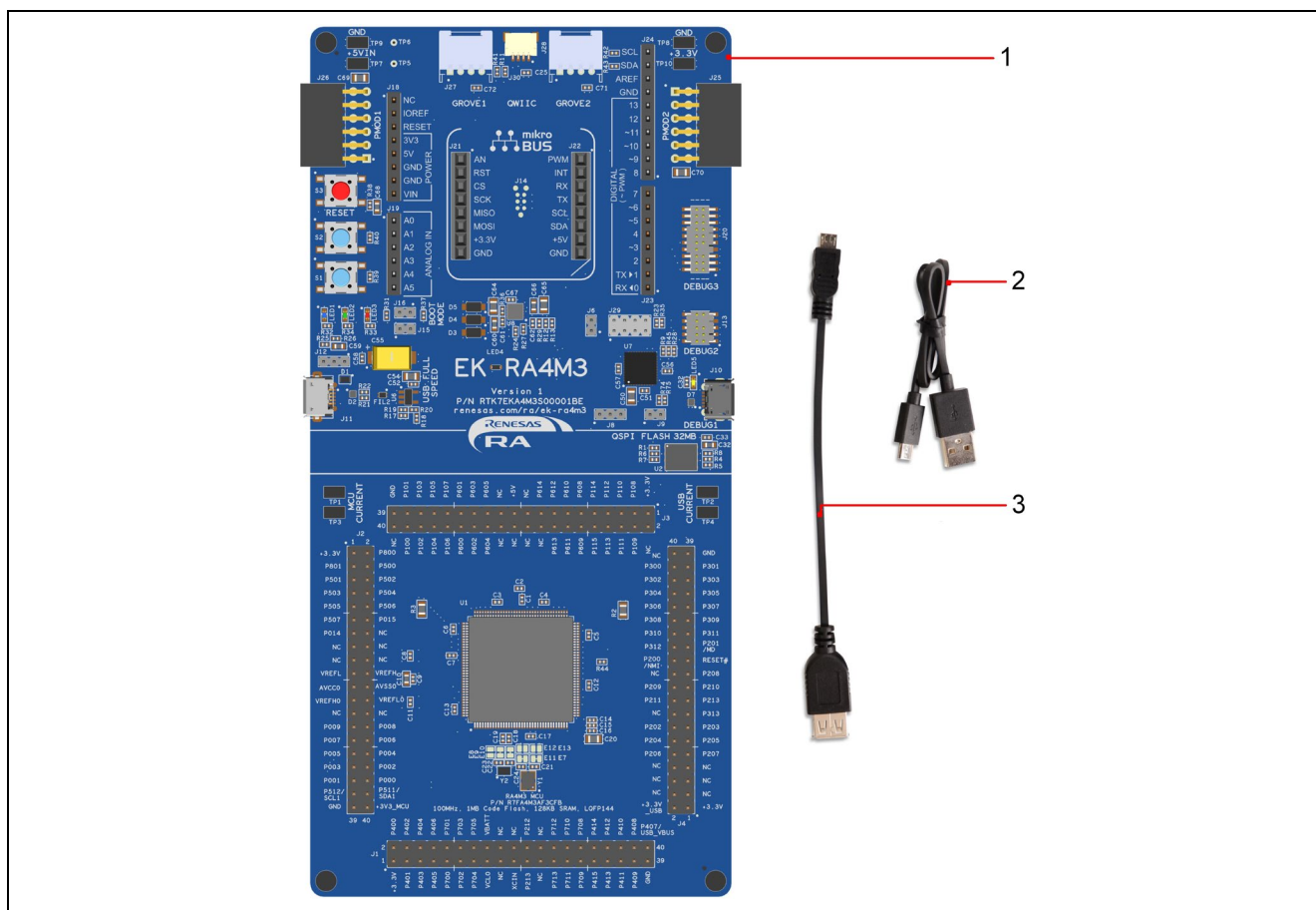
図 1 EK-RA4M3 評価キット構成
