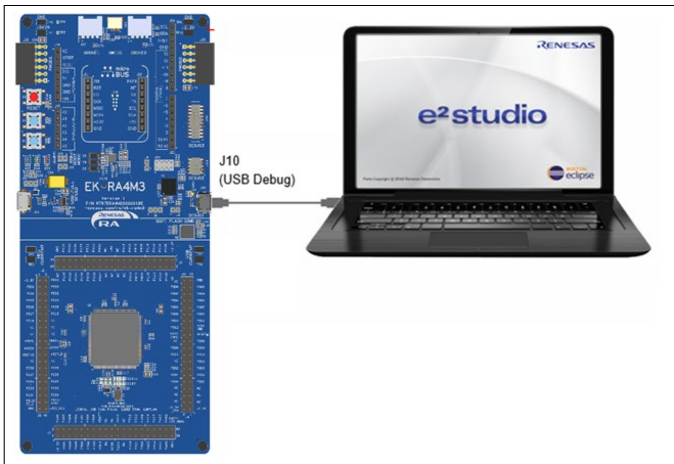
図 23 USB デバッグポートを介して EK-RA4M3 ボードをホスト PC に接続
