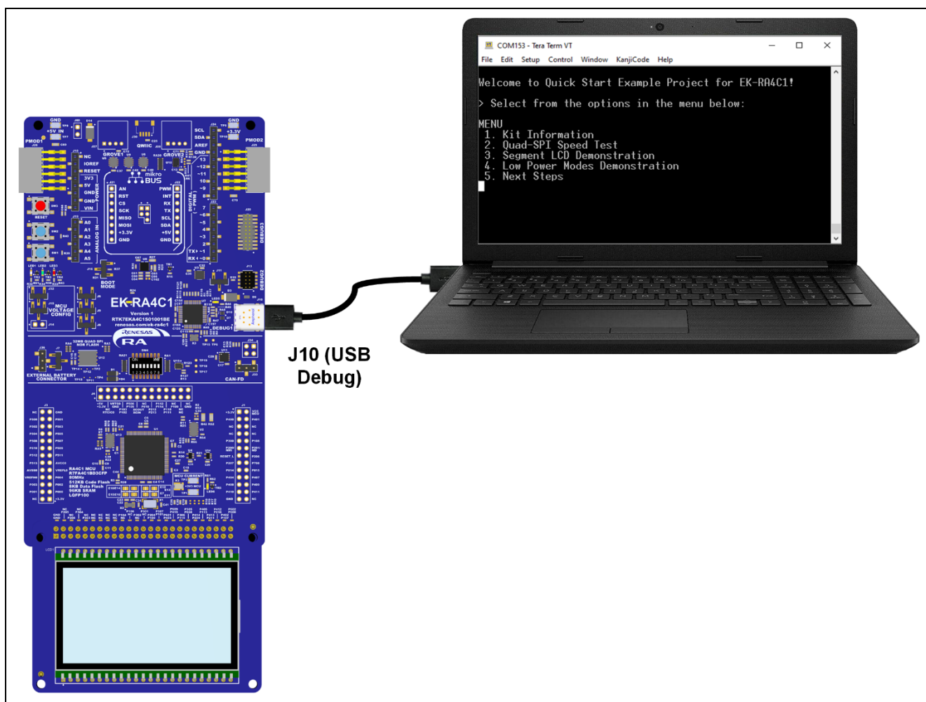
図 3. EK-RA4C1 ボードを USB デバッグ経由でホスト PC に接続
