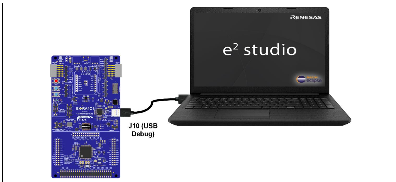
図 32. USB デバッグポートを使用した EK-RA4C1 ボードとホスト PC の接続
