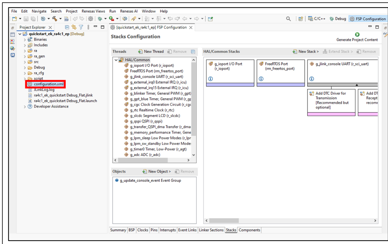
図 26. FSP Configuration ウィンドウの起動
