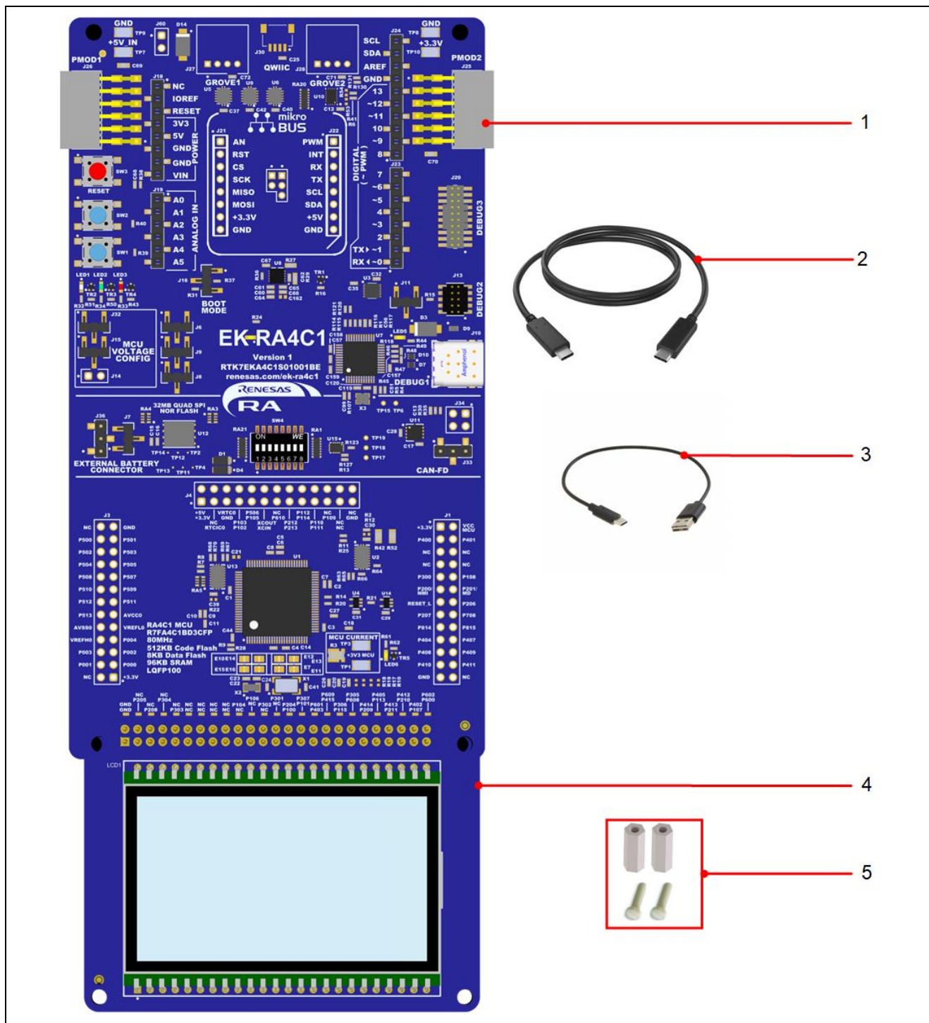
図 1. EK-RA4C1 キットの構成
