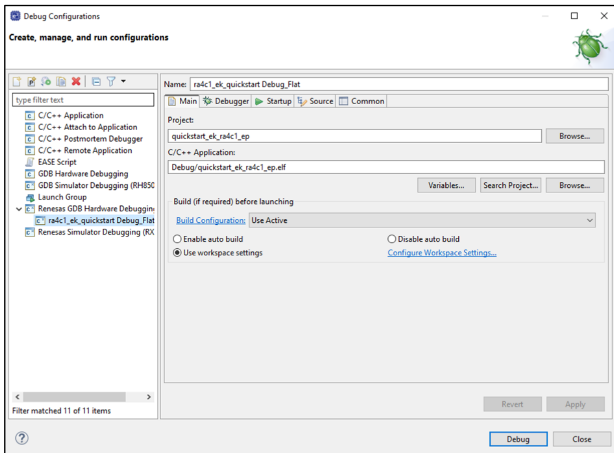
図 34. デバッグイメージの選択
